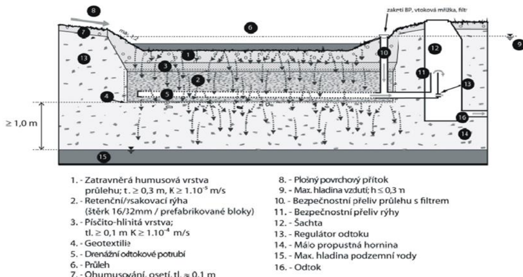
Obrázek 4: Vsakovací průleh - rýha s regulovaným odtokem (Vítek, Asio)
