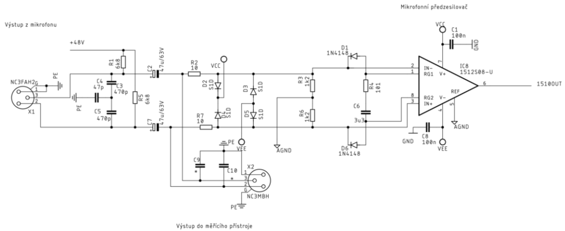
Obr. 5.3: Návrh předzesilovače.
