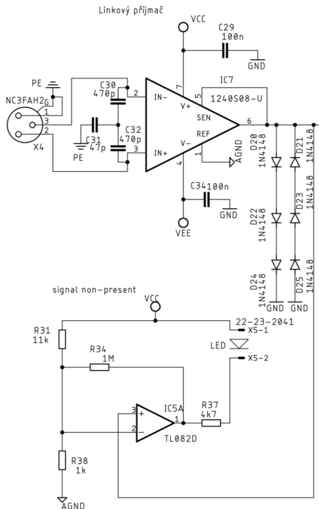
Obr. 5.4: Návrh linkového přijmače.
