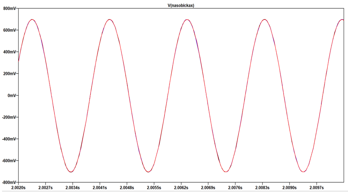
Obr. 4.7: Přibližná správně kompenzovaná simulace.
