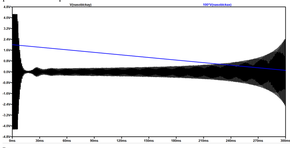
Obr. 3.2: První simulační schéma.
