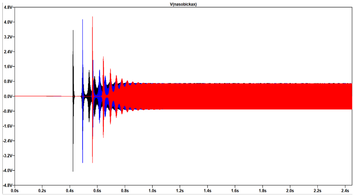
Obr. 4.6: Správně kompenzovaná simulace.
