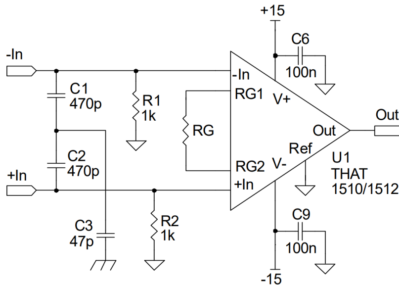
Obr. 2.5: Mikrofonní předzesilovač THAT1510.
