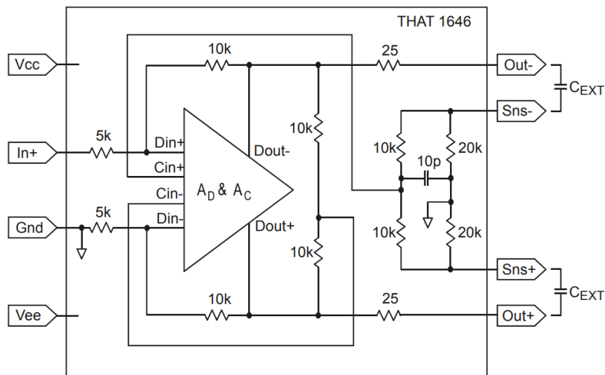
Obr. 2.4: Usměrňovač THAT1646.
