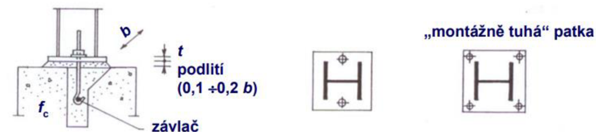
Obr. 25 Kloubové patky [20]
