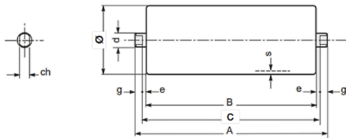
Obr. 34 Váleček PSV/I-FHD nosné stolice značky Rumelca [6]
