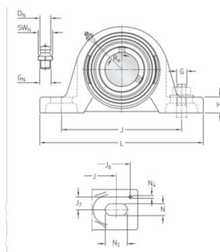
Obr. 46 Hlavní rozměry ložiskové jednotky SKF SY 40 TR [24]
