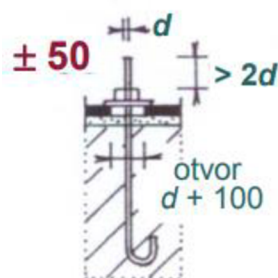
Obr. 17 Předem zabetonovaný šroub s hákem [20]
