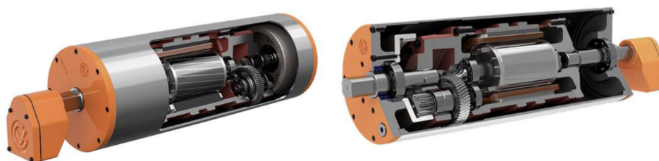
Obr. 14 Elektrobuben [14]
