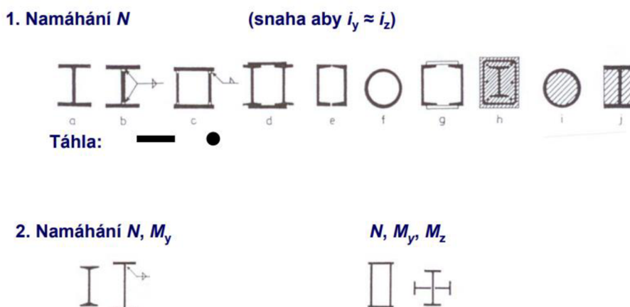
Obr. 24 Průřezy sloupů [20]
