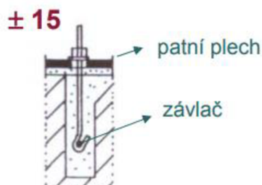
Obr. 18 Dodatečně osazený šrouby do závlače [20]
