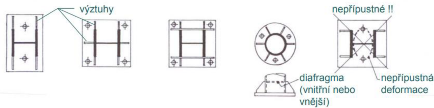
Obr. 26 Vyztužené patky [20]
