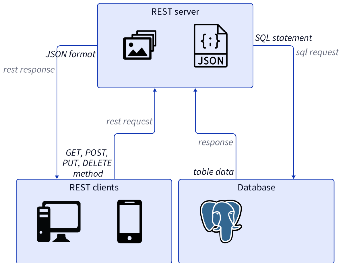
Obrázek 4: REST komunikační diagram [Vlastní tvorba]
