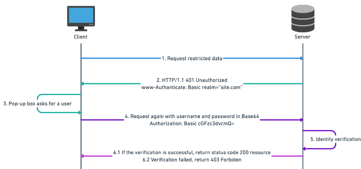
Obrázek 6: HTTP autentizace [27]
