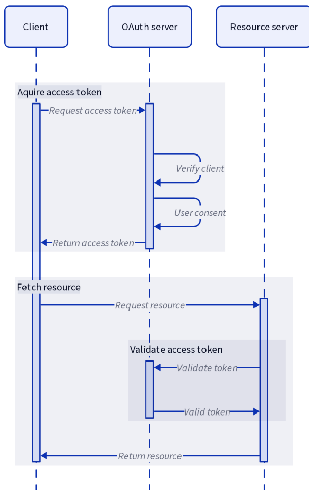
Obrázek 9: Ověření pomocí OAuth 2.0 [Vlastní tvorba]
