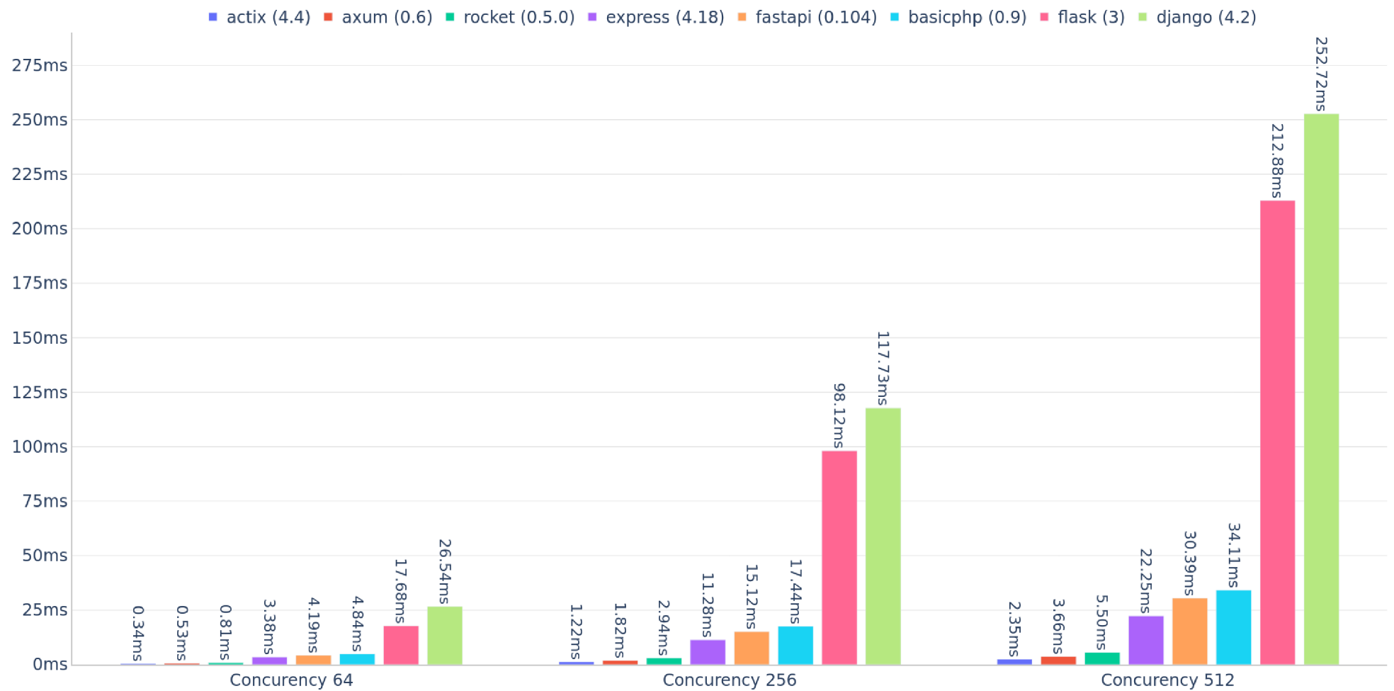
Obrázek 42: Porovnání frameworků - P75 latence [32]
