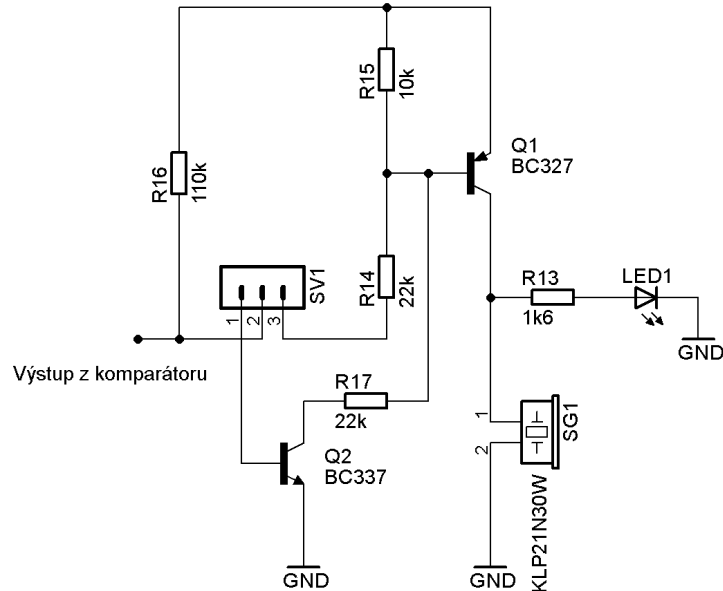
Obr. 3.10: Zapojenie signalizácie pomocou LED a sirénky
