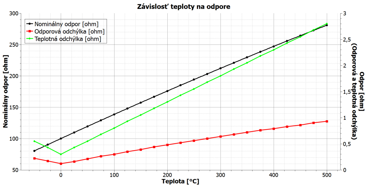
Obr. 3.3: Graf závislosti odporu na teplote, odporová a teplotná odchýlka - podľa tabuľky z [27]
