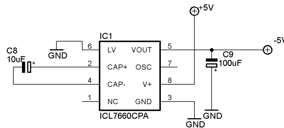
Obr. 3.12: Zapojenie napätového meniča ICL7660
