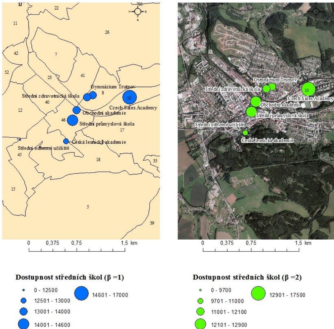
Obr. 31: Dostupnost středních škol při kritické vzdálenosti R = 15 minut (exponenciální funkce)
