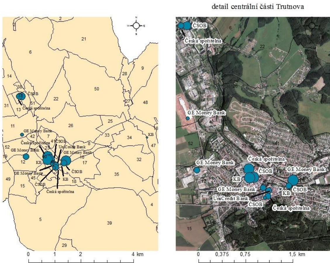
Obr. 45: Dostupnost bankomatů při kritické vzdálenosti R = 10 minut v Trutnově (exponenciální funkce)
