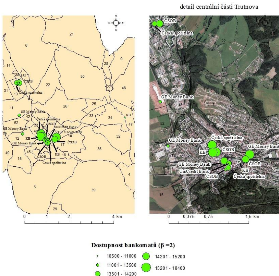
Obr. 49: Dostupnost bankomatů při kritické vzdálenosti R = 15 minut v Trutnově (exponenciální funkce)
