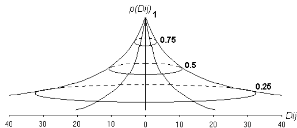
Obr. 5: Modifikovaná paretovská funkce sousedství
