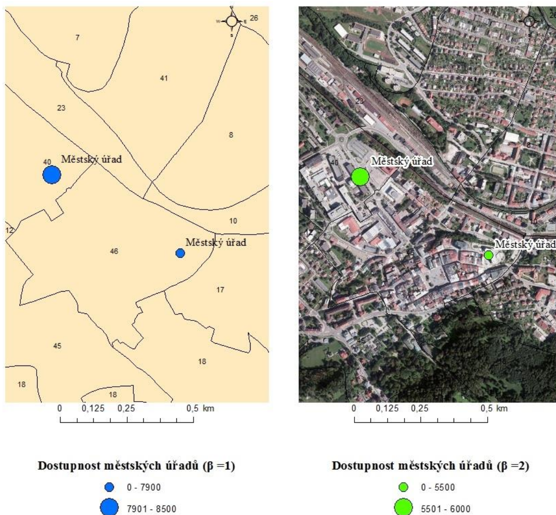
Obr. 38: Dostupnost úřadů při kritické vzdálenosti R = 795 metrů (exponenciální funkce)
