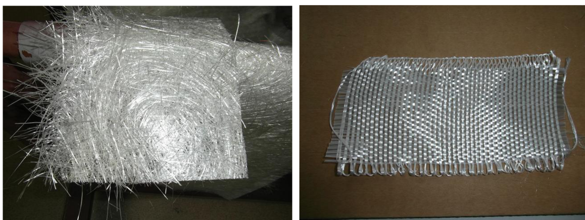
Obr. 8 Typy sklovýztuhy: skelná rohož (vlevo), rovingová tkanina (vpravo).
