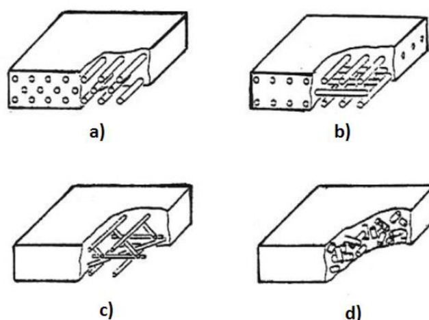
Obr. 7 Prostorové uspořádání vláken výztuže [13].
