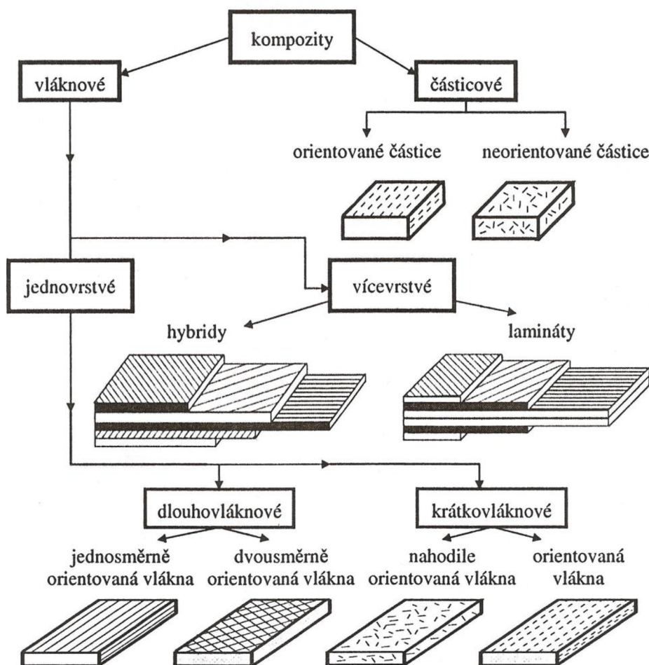
Obr. 5 Rozdělení kompozitů podle druhu výztuže [11].
