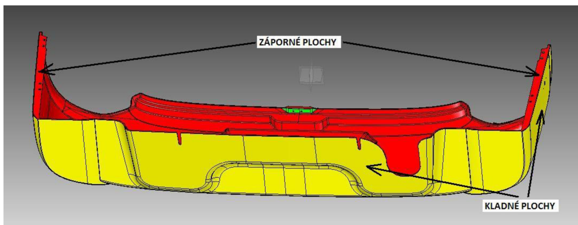
Obr. 19 Analýza úkosu ploch.
