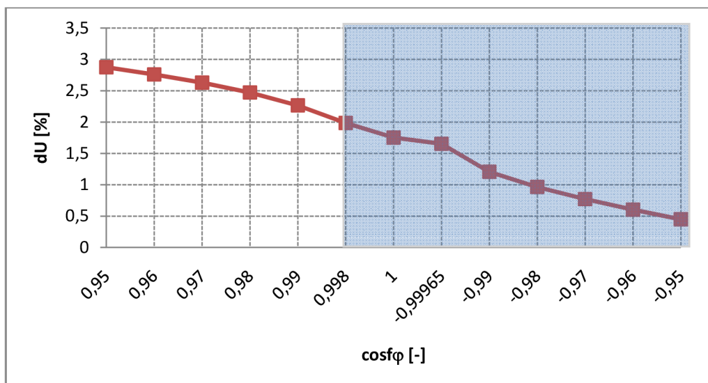
Obr. 4-5 Závislost změny napětí na účinniku VTE v místě připojení
