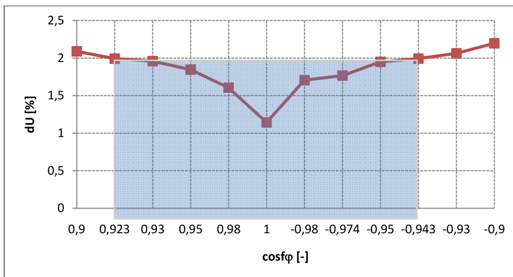
Obr. 4-9 Závislost změny napětí na účinnosti FVE v místě připojení – náhradní stav č. 2
