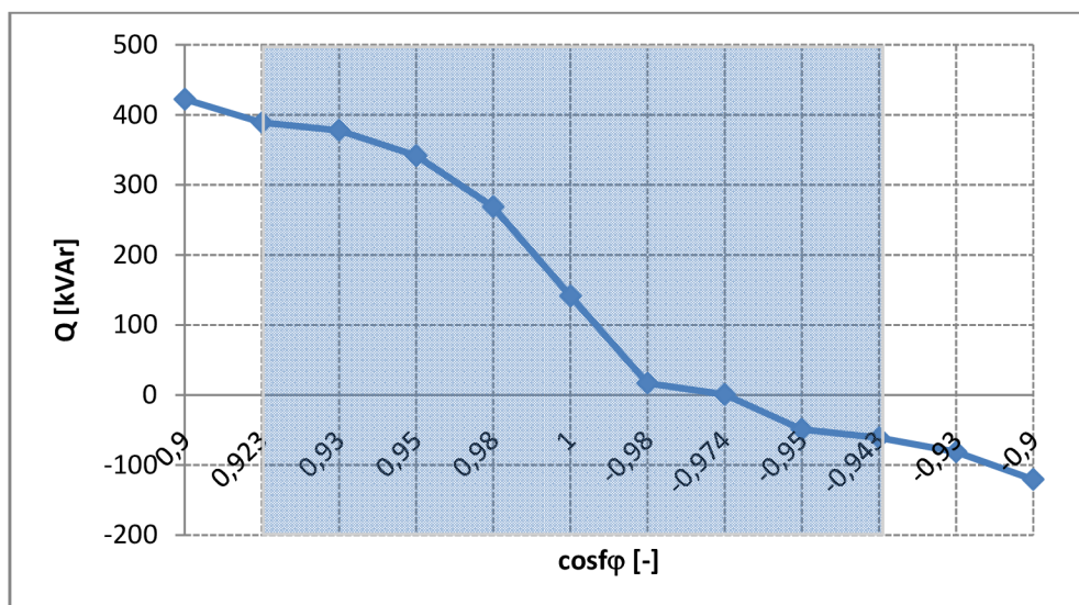
Obr. 4-8 Změna jalového výkonu v závislosti na změně účinnosti FVE v místě připojení – náhradní stav č. 2
