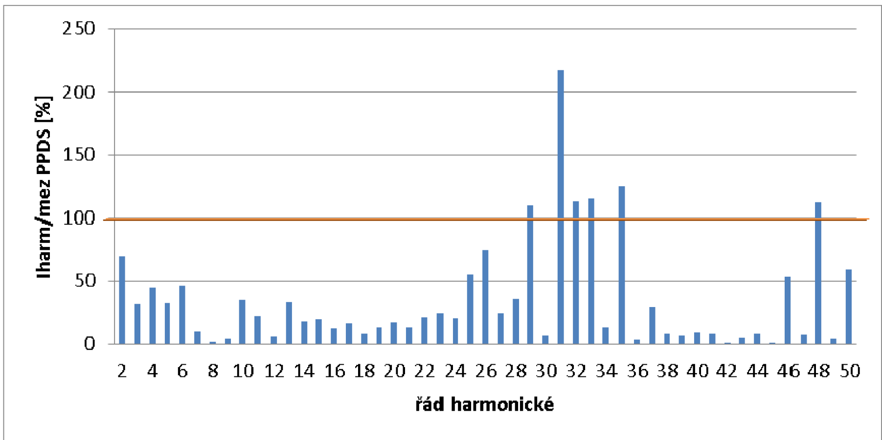
Obř. 4-13 Poměrné emise harmonických proudů
