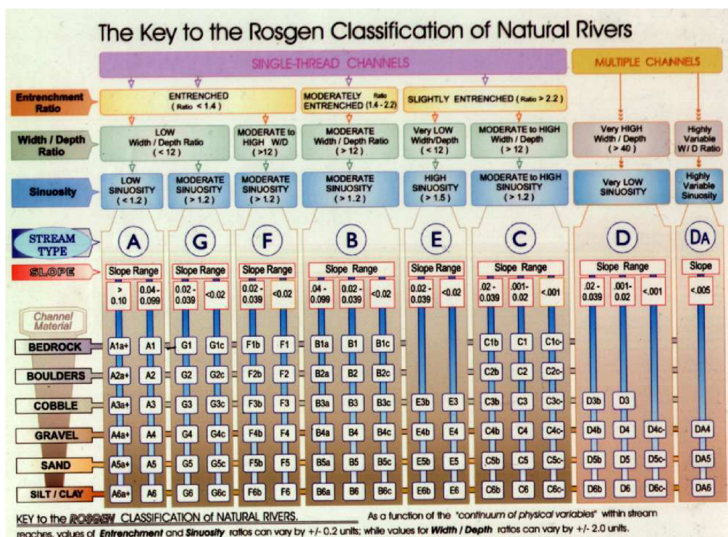
Obrázek 3: Klíč k rychlému a efektivnímu zařazení toku do metodiky dle Rosgena. Nejprve určení, jestli jde o jednonábový nebo větvičí se tok. Pak následuje stanovení poměrů rozliv/korytu, šířka/hloubka a délka toku/délka údolí. Nakonec už se rozhoduje pouze na základě sklonu a složení dnových sedimentů. Dle tohoto klíče také vzniká více než základních 41 typů, většina typů prvního stupně se v závislosti na sklonu dále rozděluje (Rosgen, 1996).
