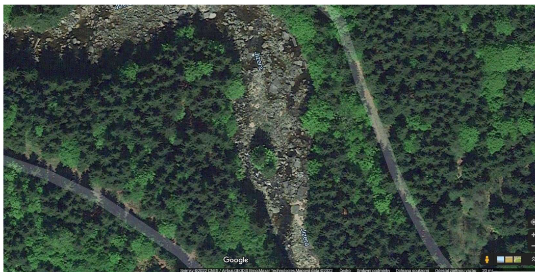
Obrázek 18: Lokalita 8: patrná kombinace stupňů a tůň. Jasně patrné jsou i rozsáhlé středové balvanité akumulace na začátku a konci oblouku, oba mírně zpevněny vegetací. Směr toku od horního ke spodnímu okraji. Zdroj: Google Maps ©2022.
