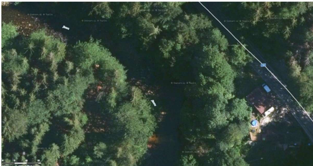
Obrázek 21: Lokalita 11: Nepřiliš zřetelný výřez ortofotomapy. Konkávní tůň a konvexní náplň tvořená valouny. Nad obloukem drobné peřeje. Směr toku od horního ke spodnímu okraji. Zdroj: Mapy.cz ©2019.
