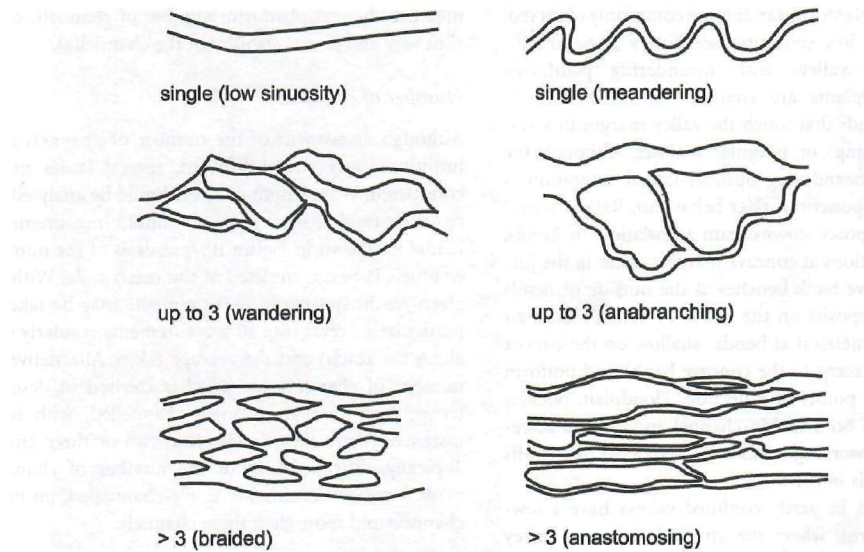
Obrázek 6: Znárodnění počtu kanálů v půdorysném zobrazení (Fryirs a Brierley, 2013).
