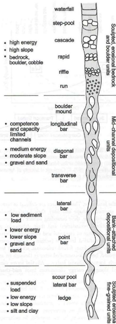
Obrázek 5: Znáornění vybraných geomorfologických tvarů v podélném profilu toku, seřazených podle energie toku a schopnosti proudu unášet sedimenty (Fryirs a Brierley, 2013).
