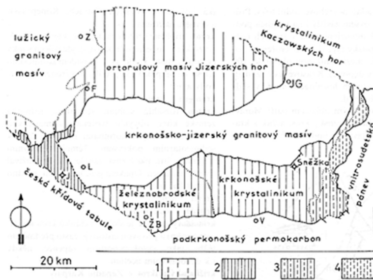
Obrázek 8: Stavba Krkonoško-jizerského krystalinika, převzato (Petránek a kol., 2016). 1 – nízká rula, 2 – ještědské krystalinikum, 3 – rýchorské krystalinikum, 4 – leszczywiecká jednotka; F – Frýdlant, J – Ještěd, JG – Jelenia Góra (Polsko), L – Liberec, V – Vrchlabí, Z – Zawidów (Polsko), ŽB – Železný Brod (Petránek a kol., 2016).
