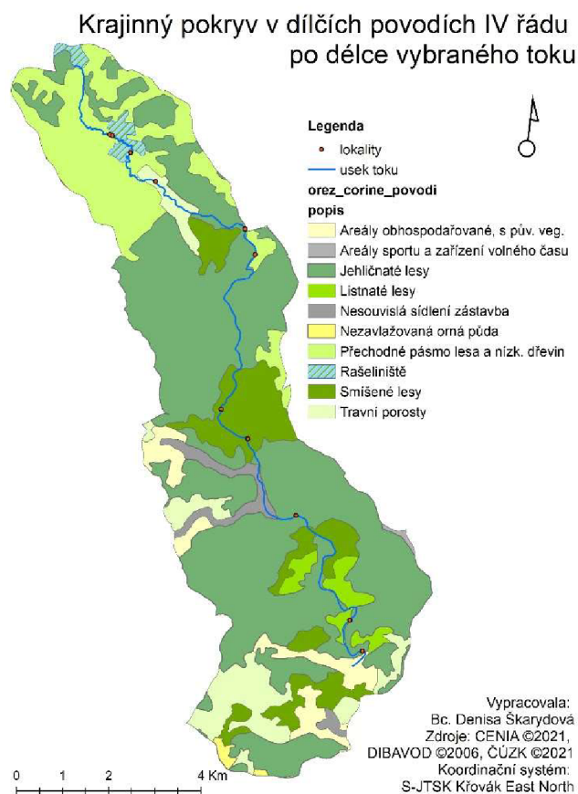
Obrázek 10: Mapa krajinného pokryvu pro povodí IV. řádu Jizerky a dotýčných povodí Jizery CENIA ©2021
