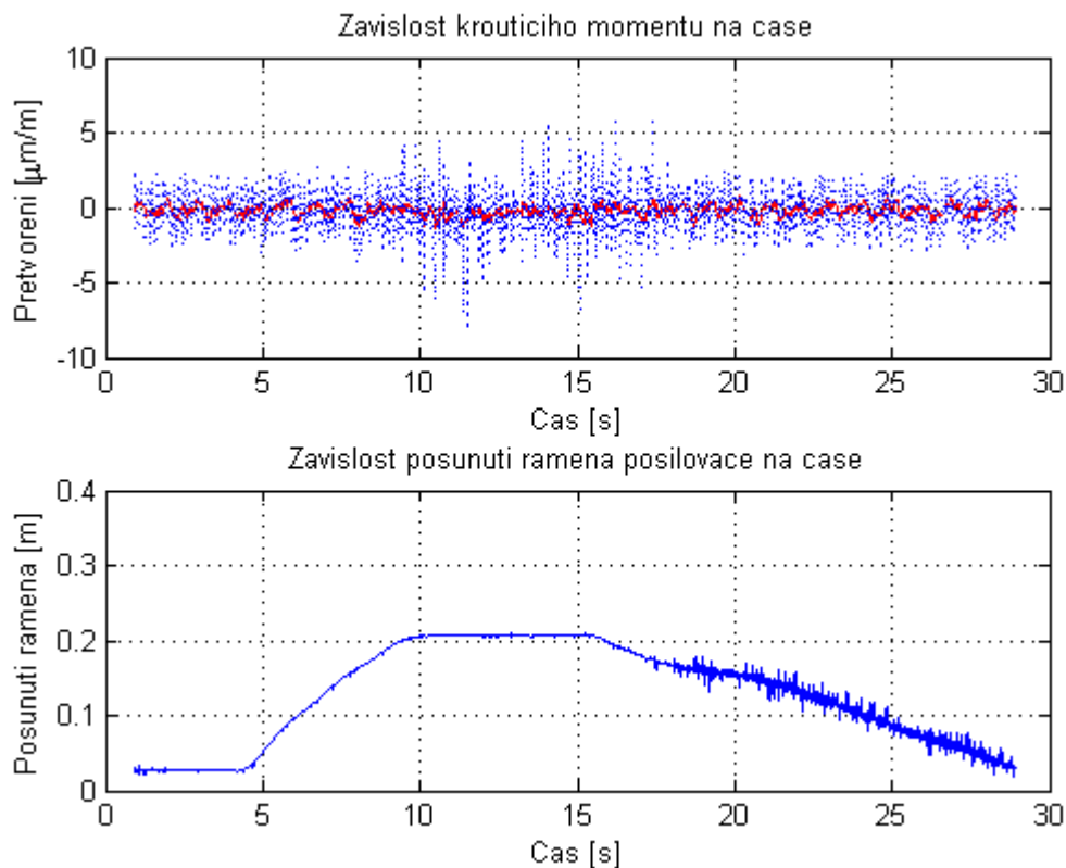
Obrázek 4.12: Graf měřených závislostí při rychlosti vozu 20km/h
