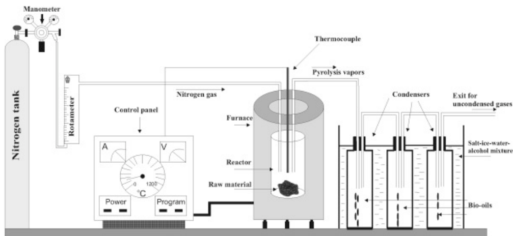
Obrázek 16 - Reaktor s pevným ložem (Aysu et al., 2014)
