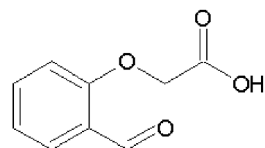
Obrázek 30: Strukturální vzorec kyseliny 2-formylphenoxyoctové.
