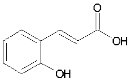
Obrázek 36: Strukturální vzorec kyseliny 2-hydroxyskořicové.
