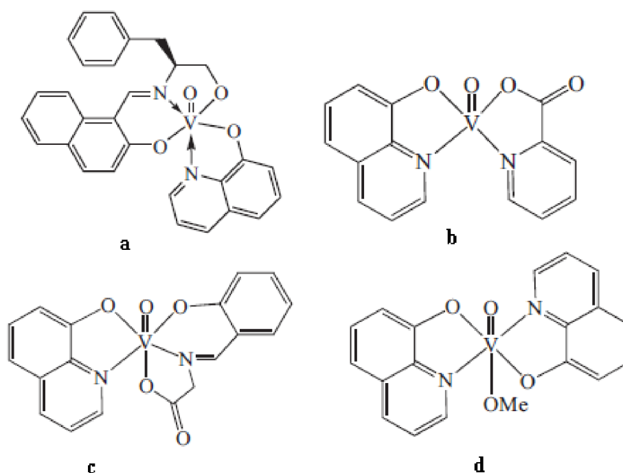
Obrázek 17: Strukturální vzorce sloučenin a-d. (51)
