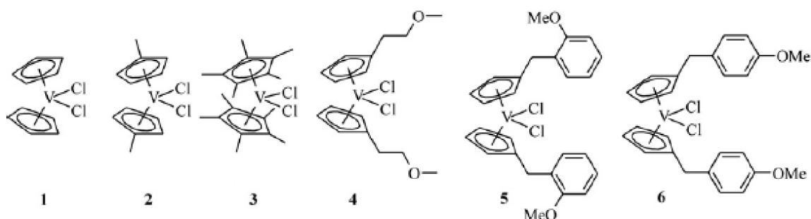
Obrázek 3: Strukturální vzorce vanadocenu. (21)
