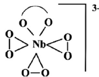
Obrázek 23: Strukturální vzorec aniontu [Nb(Asc)(O_2)_3] .
