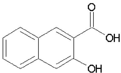
Obrázek 37: Strukturální vzorec kyseliny 3-hydroxy-2-naftoové.
