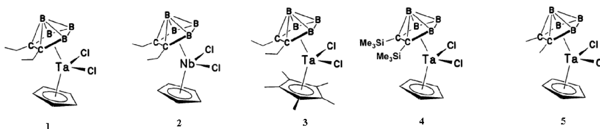
Obrázek 25: Struktura metalokarboranů tantalů a niobu
