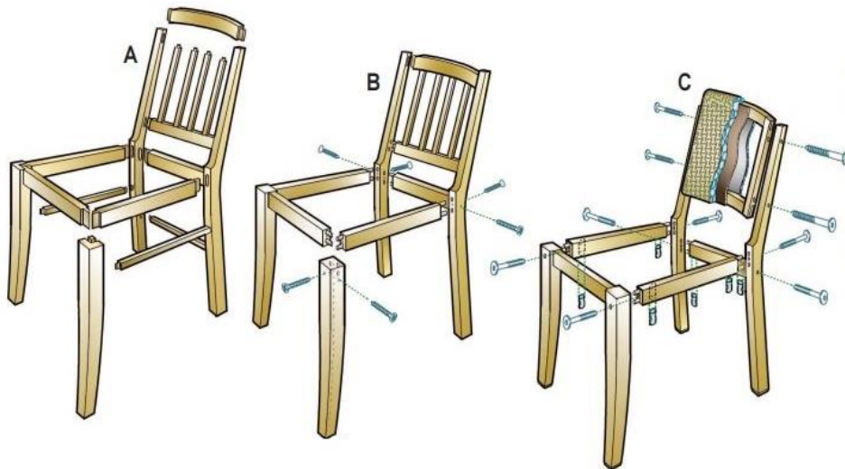
Obrázek 7: Spoje dílců židli tvarovaných třískovým obráběním
