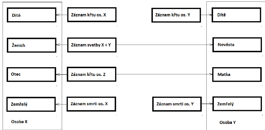
Obrázek 3.3: Diagram Identity modelu aplikace Moragen.
