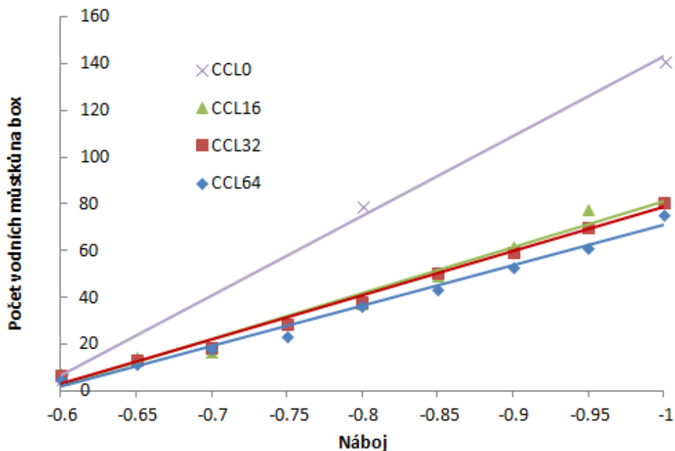
Obr. 28: Vliv počtu vodních můstků na náboji pro síť s různým stupněm kovalentního zesílení
