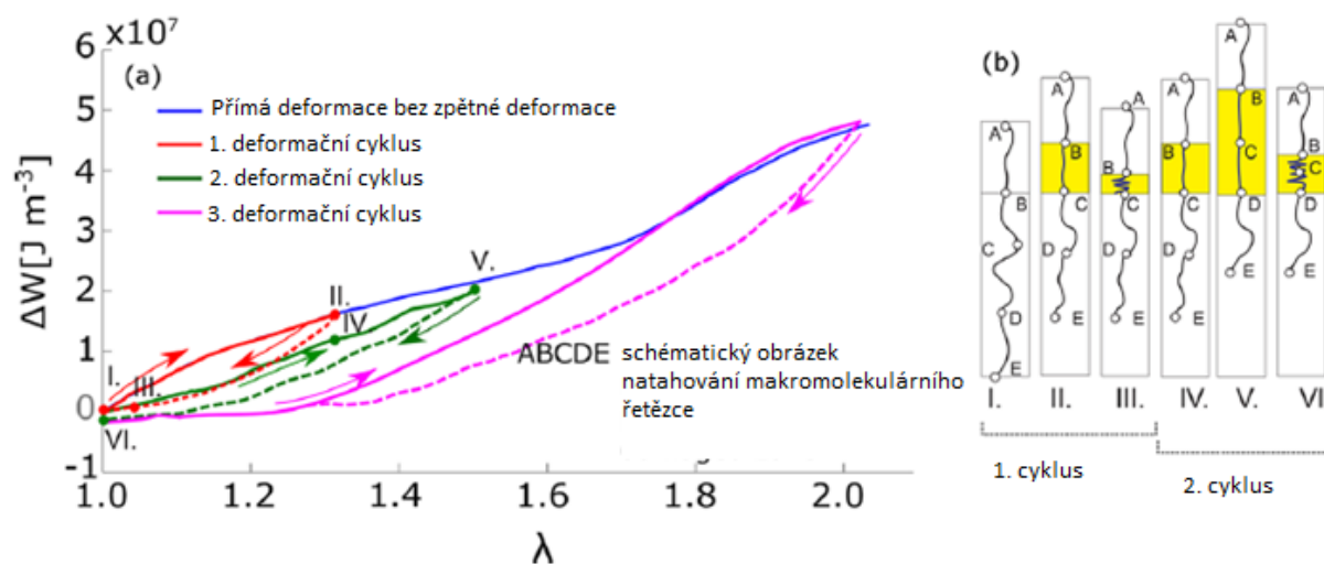
Obr. 10: a) Deformační odezva modelu fyzikálního gelu během vícenásobného deformačního namáhání (Mullinsův efekt). Plné čáry značí přímou deformaci, čárkované zpětnou deformaci. b) Natahování řetězového segmentu A-B-C-D-E, žlutě je zvýrazněna část, která podléhá poškození.
