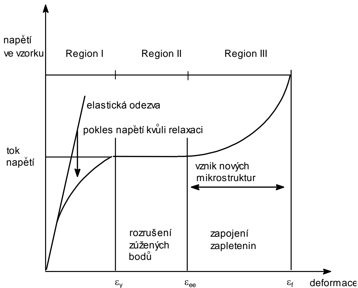
Obr. 7: Klasifikace deformační "stress-strain" křivky do tří regionů
