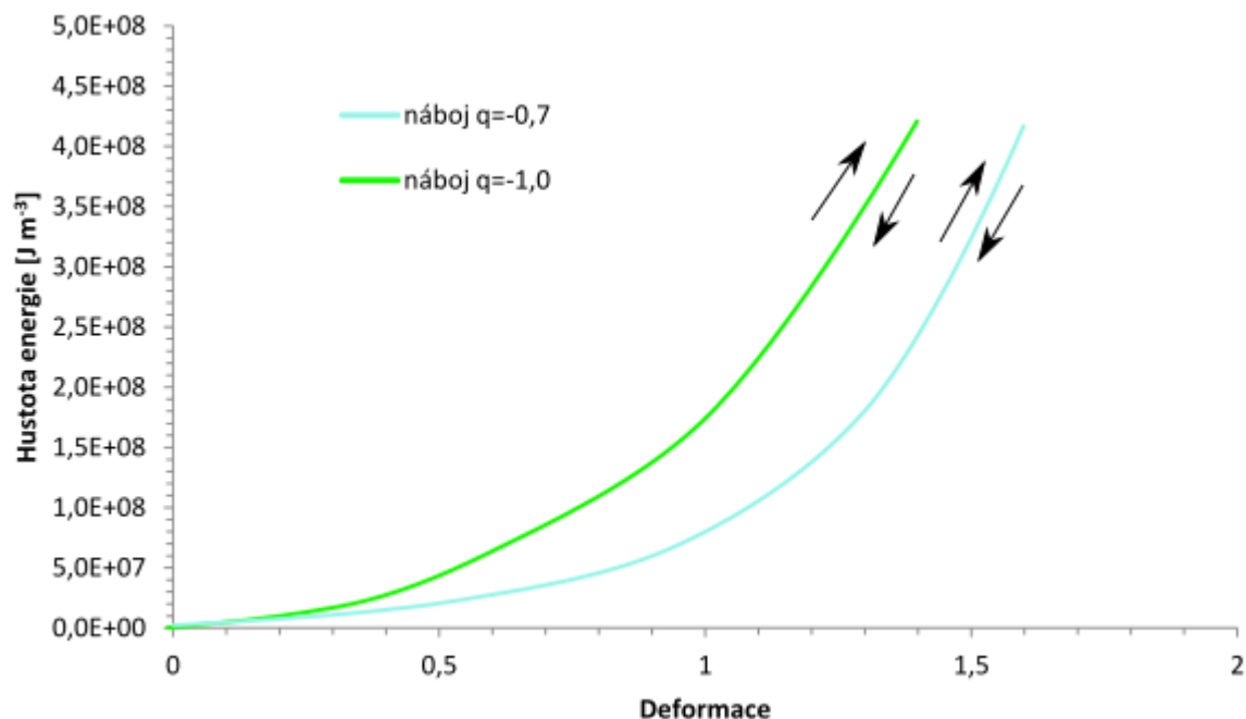
Obr. 20: Hybridní kovalentní (64 CCL na box) a iontové sítě. Kovalentní síť s nízkým nábojem (náboj q = -0,7 e tyrkisová křivka) a kovalentní síť s vysokým nábojem (náboj q = -1,0 e světle zelená křivka) vykazovaly zcela elastickou odezvu.
