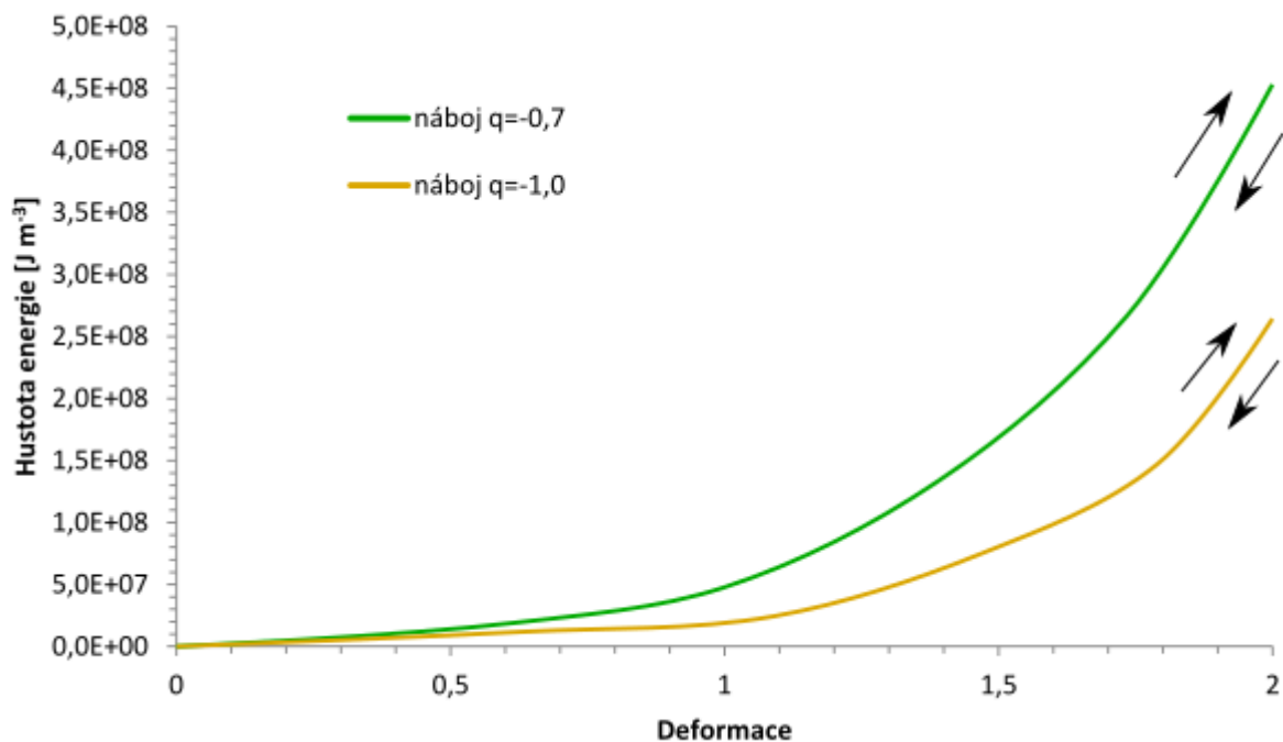
Obr. 19: Hybridní kovalentní (32 CCL na box) a iontové sítě. Kovalentní síť s nízkým nábojem (náboj q = -0,7 e a oranžová křivka) a kovalentní síť s vysokým nábojem (náboj q = -1,0 e a zelená křivka) vykazovaly již elastickou odezvu.
