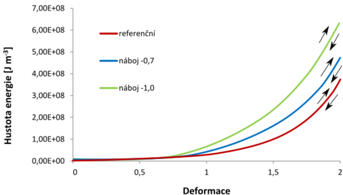
Obr. 27: Deformační křivky pro síť s kovalentním zesítěním 64 CCL na box. Jako referenční křivka byla zvolena binární fyzikálně-kovalentní síť (červená křivka). Postupně se zvyšoval náboj: q = -0,7 e (modrá křivka), q = -1,0 e (zelená křivka). S rostoucím nábojem se zvyšovala tuhost sítě.
