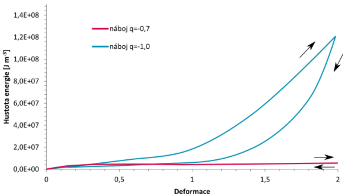
Obr. 18: Hybridní kovalentní (16 CCL na box) a iontové sítě. Kovalentní síť s nízkým nábojem (náboj q = -0,7 e a červená křivka) nevykazovala takřka žádnou mechanickou odezvu. Kovalentní síť s vysokým nábojem (náboj q = -1,0 e a modrá křivka) odhalila při zpětné deformaci hysterezi.
