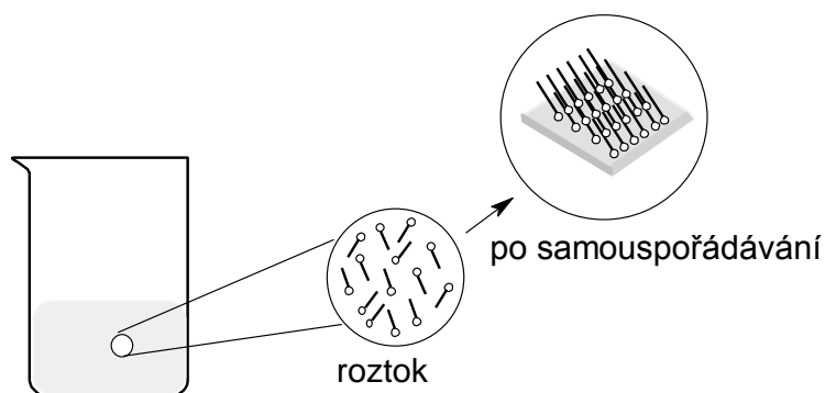
Obr. 2: Ilustrační schéma samouspořádání (self-assembly)
