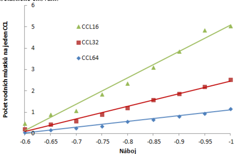
Obr. 29: Počet vodních můstků na jeden CCL v závislosti na náboji a kovalentním zesílení
