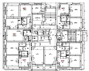
Obr. 15 Načtený půdorys
