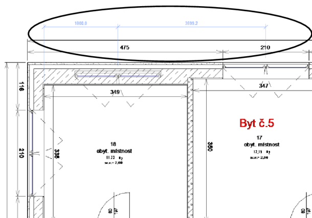
Obr. 146 Vynášecí kóty
