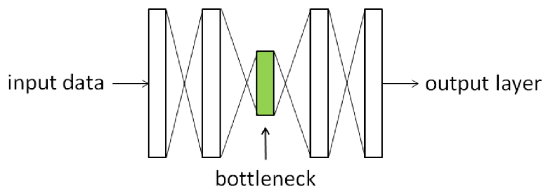
Obrázek 2.2: Neuronová síť s vrstvou s menší dimenzionalitou [23]
