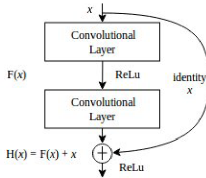
Obrázek 10.1: ResNet blok [44]
