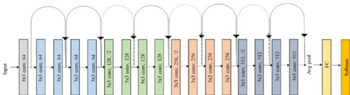
Obrázek 10.2: ResNet18 návrh [45]
