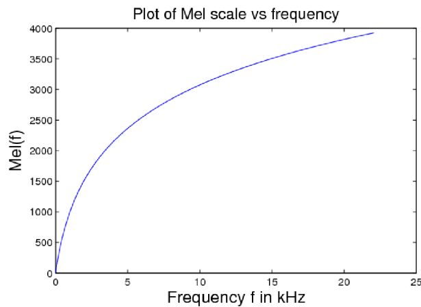
Obrázek 2.1: Mel křivka [18]
