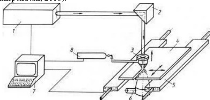
Obrázek 3 Schéma zařízení pro řezání laserem (www.mmspektrum.com)
