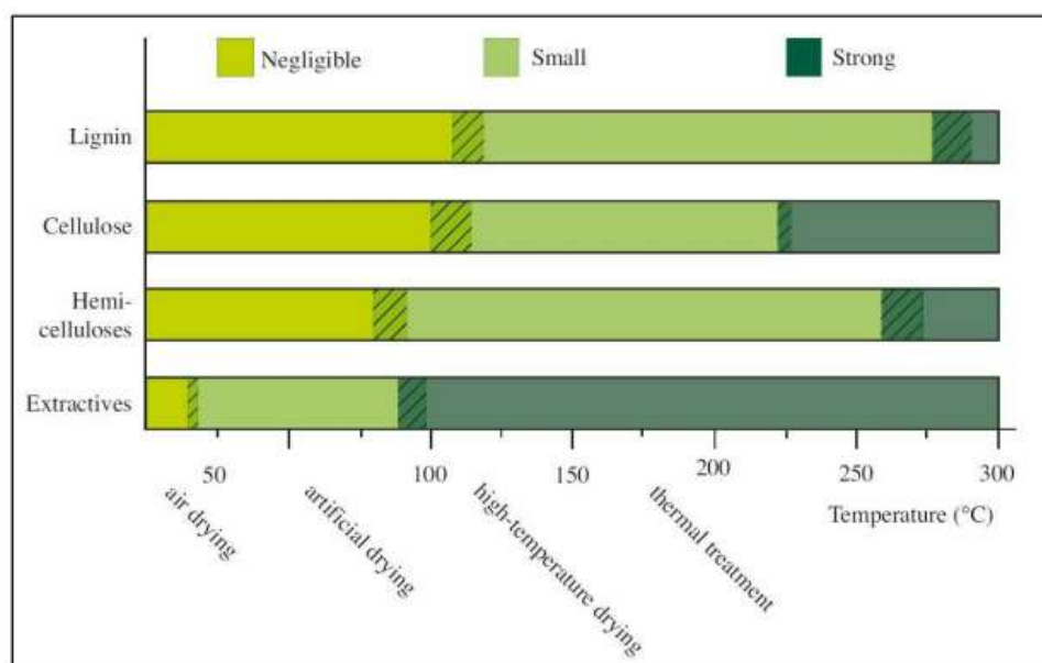
Obrázek 8 Degradace dřevních složek podle velikosti tepla (Sandberg, 2011)
