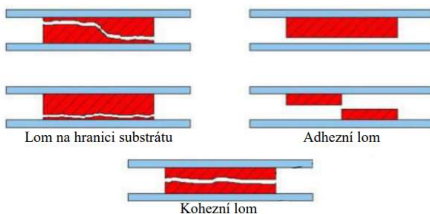
Obrázek 19 Lomy lepeného spoje (Doubek, 2014)
