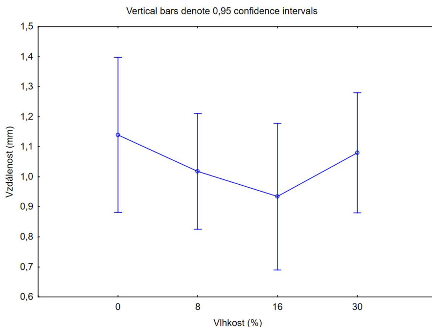
Obrázek 25 Vliv vlhkosti obráběných vzorků na protažení lepeného spoje bez statistické významnosti
