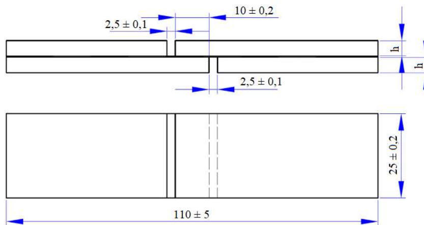
Obrázek 20 Rozměry zkušebního vzorku pro měření smykové pevnosti. (Gaff, 2020)
