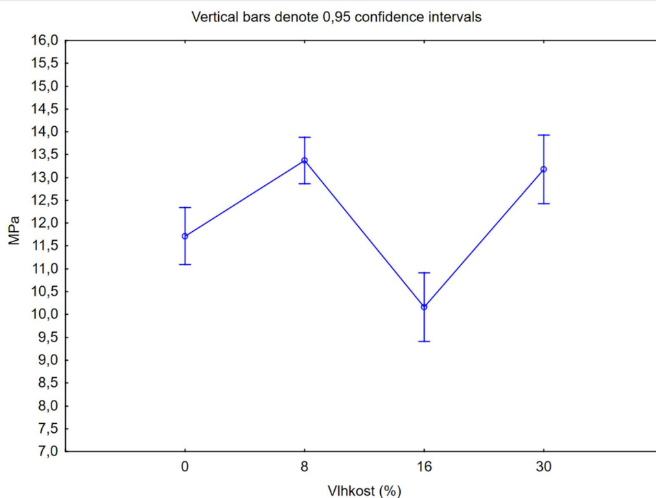
Obrázek 24 Vliv vlhkosti při řezání na smykovou pevnost lepeného spoje Porovnání protažení lepeného spoje
