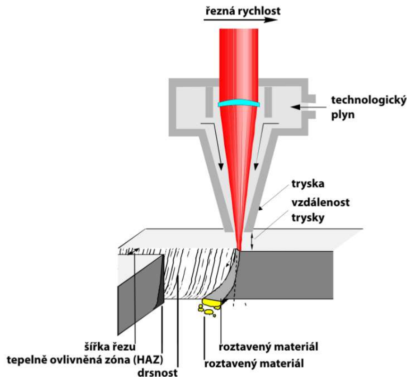
Obrázek 4 Ovlivnitelné nastavení laserového paprsku (lao.cz)
