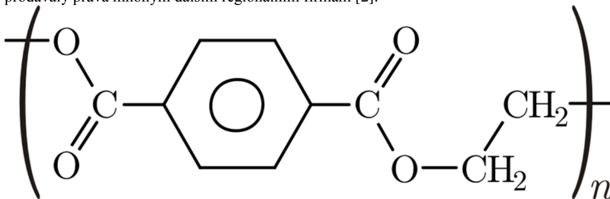
Obr. 1 Struktura polyethyltereftalátu
