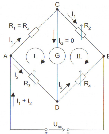
Obrázek 2.10: Zapojení Wheatstoneova můstku s odpory (Elektrotechnická měření, 2002)
