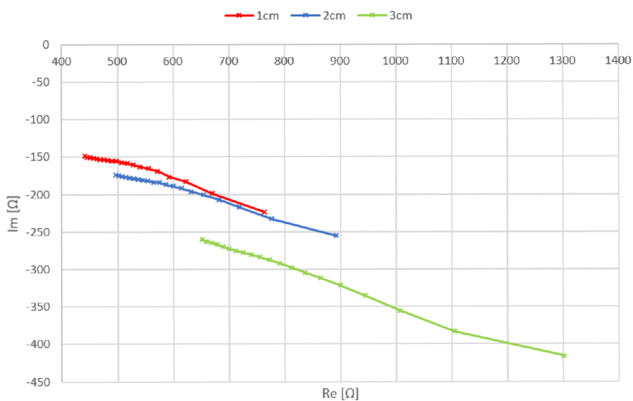
Obrázek 3.10: Metoda tří voltmetrů - impedance v komplexní rovině
