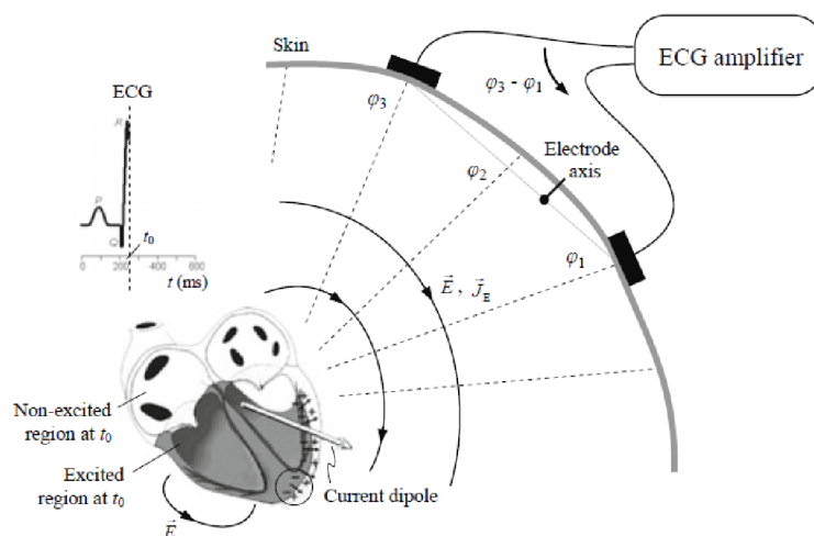
Obrázek 2.5: Elektrické pole v okolí srdce (Kaniusas, 2019, upraveno).
