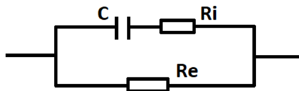
Obrázek 2.6: Cole-Coleův model elektrických vlastností tkáně (Lopot, 2016).
