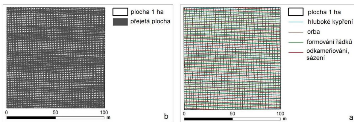
Obr. 16: Záznam trajektorie jízd (a) a stop pneumatik (b) při zakládání porostu brambor
