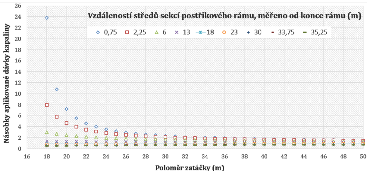
Graf 2: Nárůst/pokles dávky postříkové kapaliny v zatáčkách s rozdílnými poloměry
