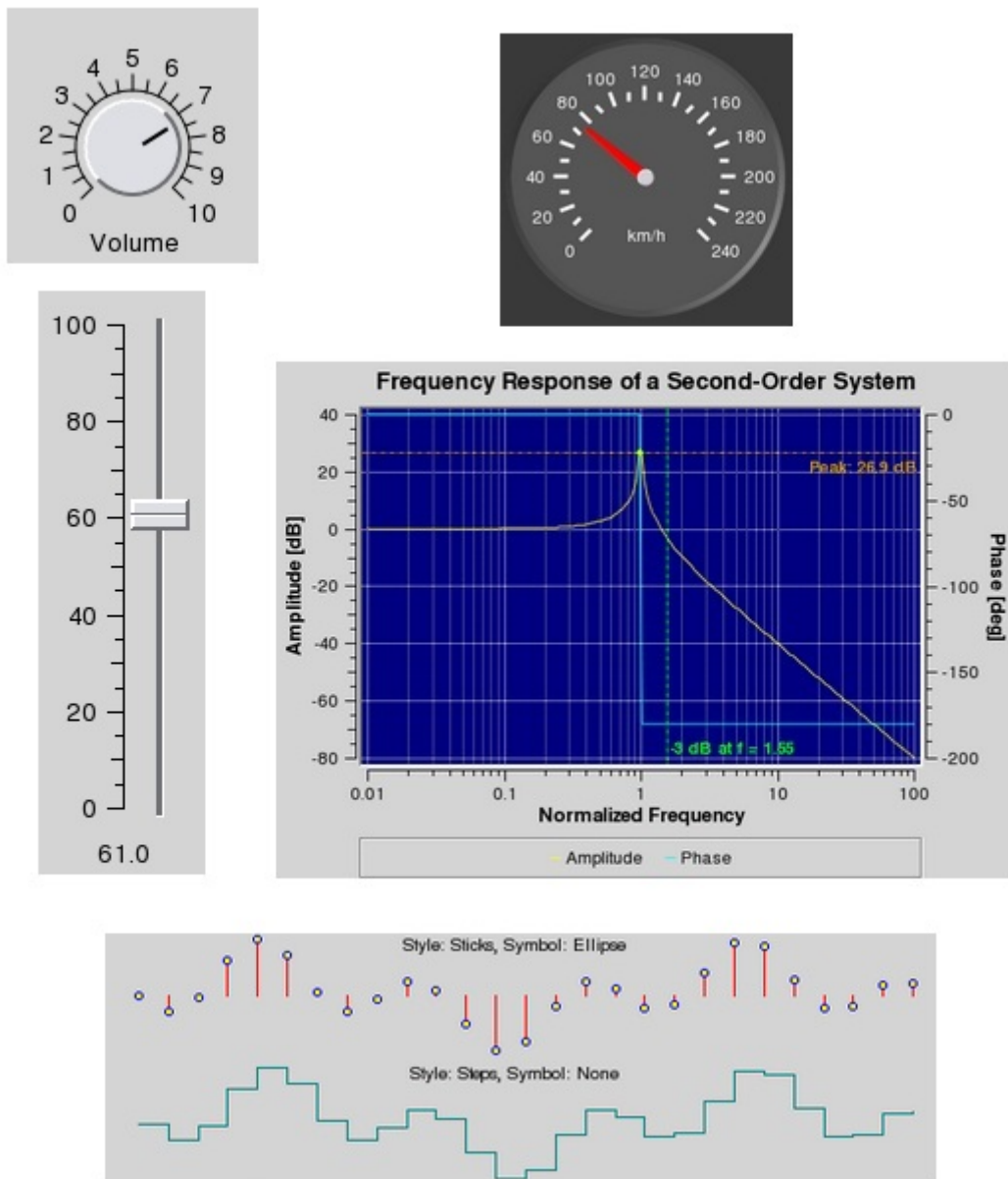
Obrázek 2.2: Ovládací prvky z knihovny Qwt
