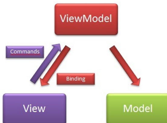
Obrázek 1.2: MVVM model[3]
