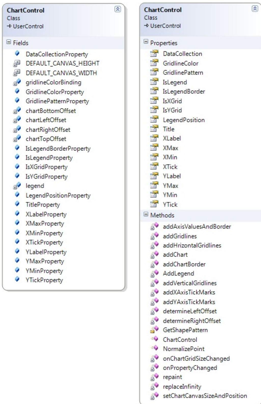
Obrázek 3.9: Třída ChartControl1
