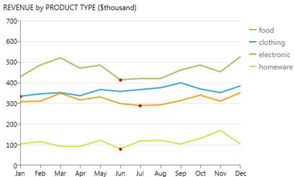
Obrázek 2.1: Telerik ChartView
