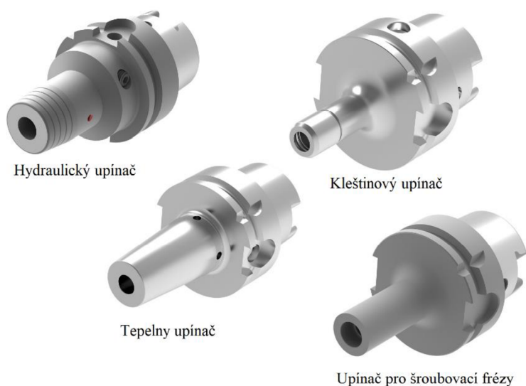
Obr. 60: - Typy nástrojových upínačů firmy WNT
