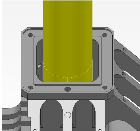
Obr. 18: Předvrtání pravoúhlé kapsy
