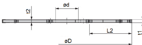
Obr. 56: Schéma rozměrových parametrů kotoučové frézy s VBD firmy WNT ([14], upraveno)
