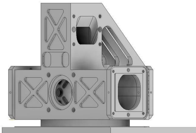
Obr. 39: Lehce odlomitelná „podříznutá“ součást
