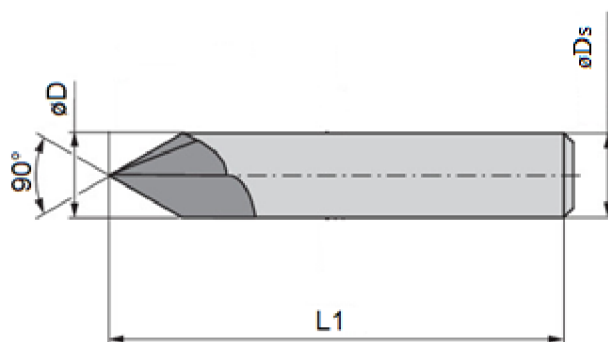
Obr. 55: Schéma rozměrových parametrů NC srážeče firmy WNT ([14], upraveno)
