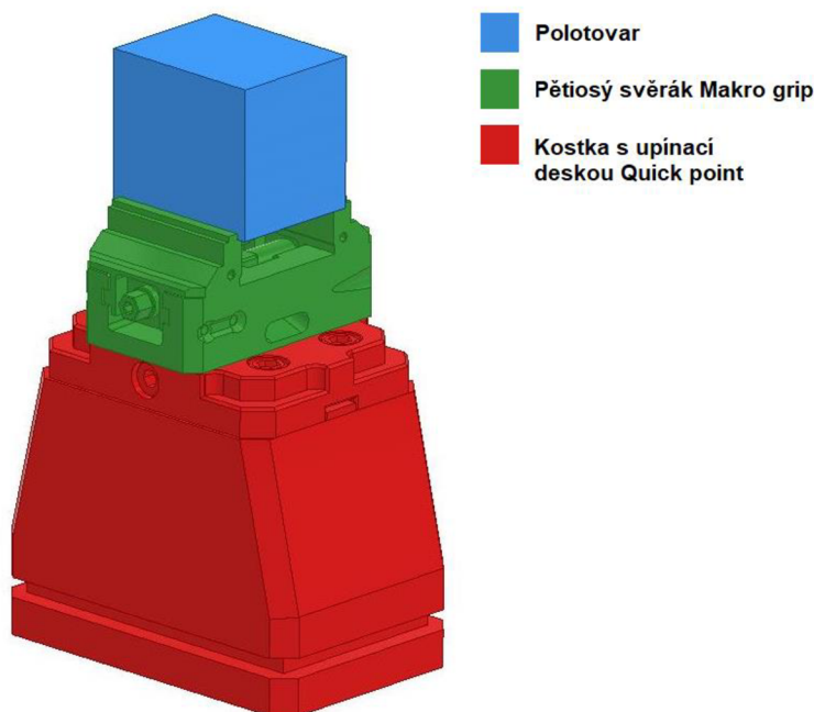
Obr. 15: Upínací sestava včetně polotovaru součástí
