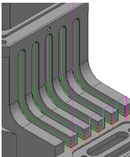
Obr. 47: Víceosé simultánní dokončení drážek
