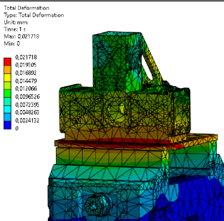
Obr. 66: Deformace součásti vlivem HSC hrubování
