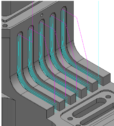
Obr. 46: Víceosé simultánní hrubování drážek zanoření pod úhlem
