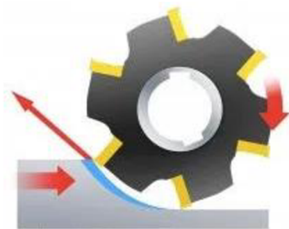
Obr. 11: Schéma nesousledného frézování [11]
