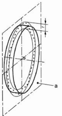
Obr. 13) Definice tolerančního pole kruhovitosti [10]
