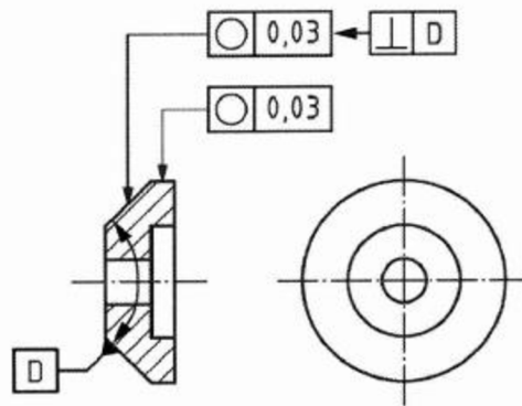
Obr. 12) Indikace kruhovitosti [10]
