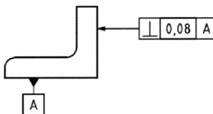
Obr. 16) Indikace kolmosti [10]
