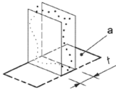
Obr. 17) Definice tolerančního pole kolmosti [10]
