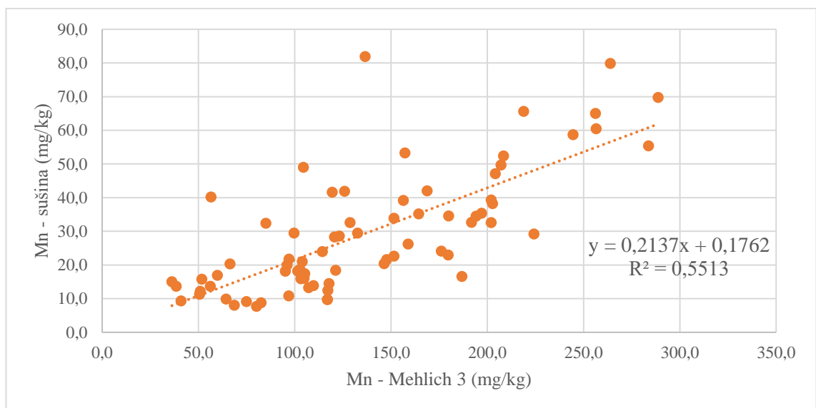
Graf 18: Regresní vztah množství manganu v sušince rostlin s manganem v půdě stanoveným metodou Mehlich 3 ( n=73 )
