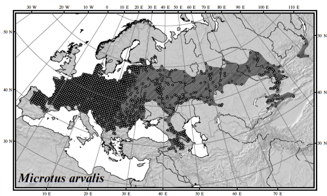
Obr. 1 Rozšíření hraboše polního v Evropě. Zdroj: Shenbrot a Krasnov (2005)
