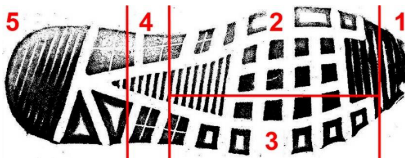
Obr. 5 – Rozdělení podešve obuvi do pěti sektorů (1 - špička, 2 - podpalcová část plosky, 3 - podmalíková část plosky, 4 – klenek, 5 - pata)
