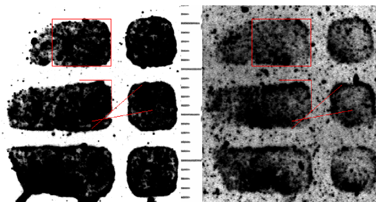
Obr. 25 – Geometrická konstrukce
