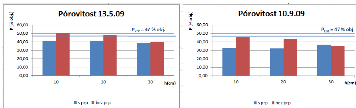
obr. č.18. Průběh pórovitosti ze dne 13. 5. 09 a 10. 9. 09
