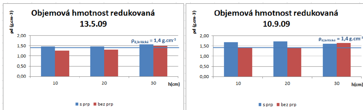
obr. č.15. Průběh objemové hmotnosti redukové ze dne 13. 5. 09 a 10. 9. 09
