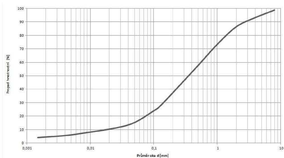
obr. č.2. Křivka zrnitosti (zdroj internet)
