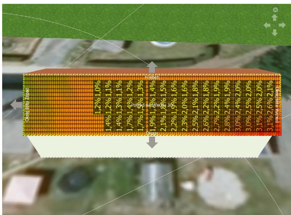
Obrázek 7-3 Vliv stínění okolních objektů fotovoltaické elektrárny
