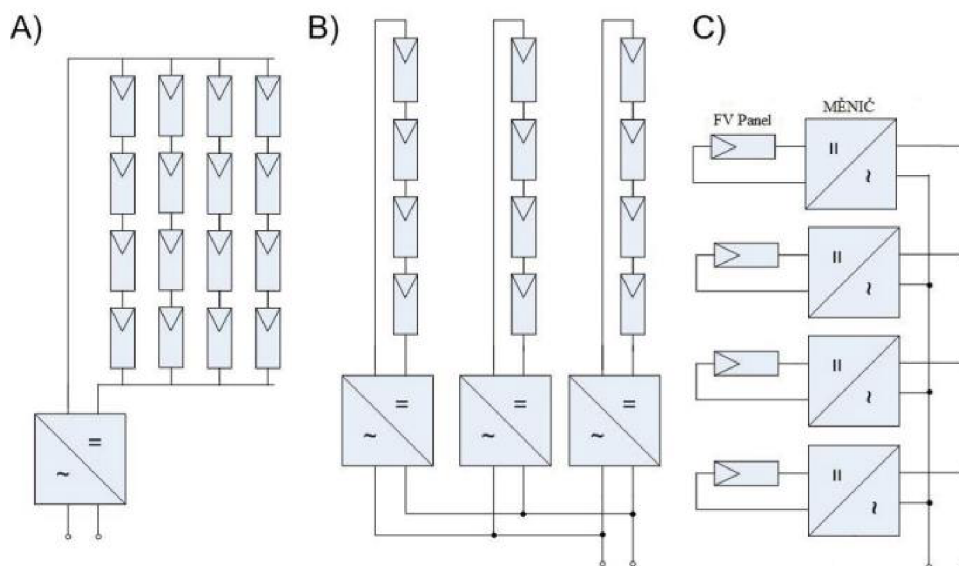
Obrázek 3-5 A) Centrální střídač B) Řetězcové (stringové) střídače C) Modulové střídače [21]
