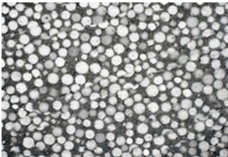
Obrázek 8: Struktura polystyrenbetonu [19].
