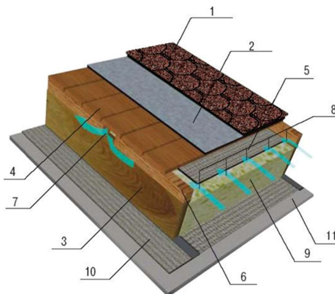
Obrázek 30: Skladba střešního pláště pomocí asfaltových šindelů – asfaltový šindel (1), podkladní pás (2), krokve (3), dřevěné bednění (4), pojistná HI (5), kontralatě (6), mezera mezi kontralatěmi (7), vzduchová mezera (8), tepelná izolace (9), parotěsná zábrana (10), sádkarton (11) [67].
