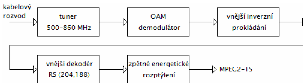
Obr. 3.2: Blokové schéma přijímače DVB-C
