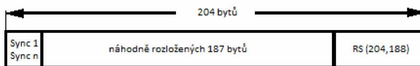
Obr. 3.4: Paket transportního toku za obvodem RS (204,188)
