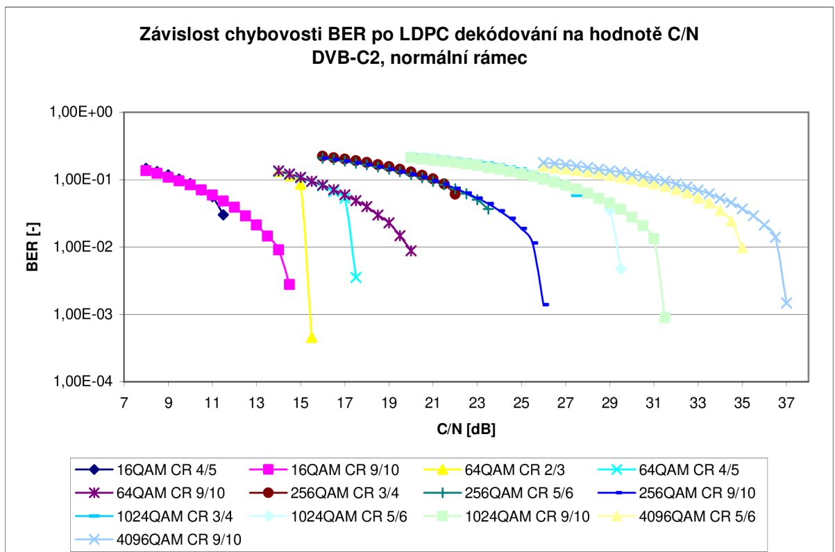
Obr. 8.5: Graf závislosti chybovosti BER po LDPC dekodování na hodnotě C/N v systému DVB-C2, normální FEC rámec
