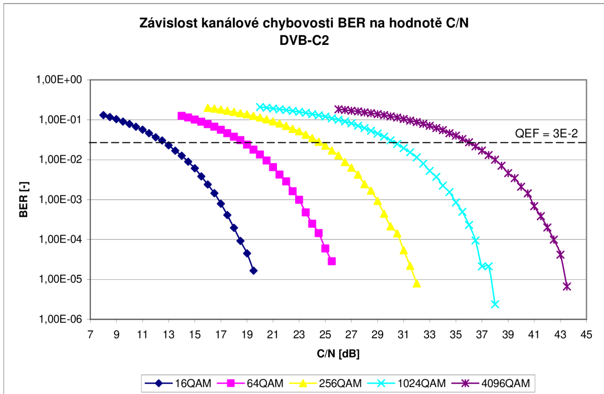
Obr. 8.2: Graf závislosti kanálové chybovosti BER na hodnotě C/N v systému DVB-C2
