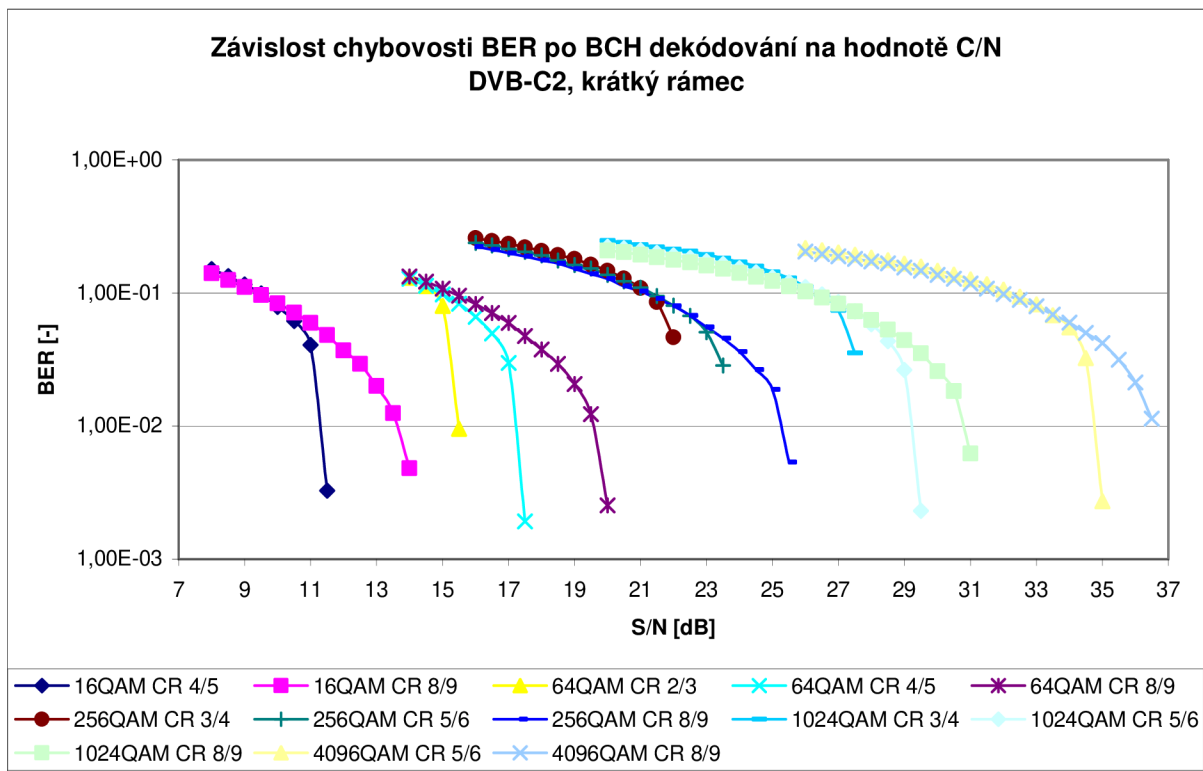
Obr. 8.4: Graf závislosti chybovosti BER po BCH dekodování na hodnotě C/N v systému DVB-C2, krátký FEC rámec
