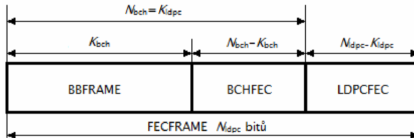
Obr. 4.5: FECFrame formát
