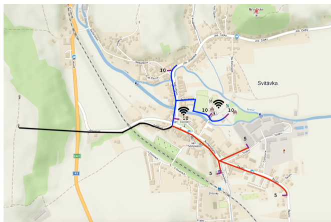
Obr. 8.1: Mapa návrhu rozšíření optické sítě v městysu Svitávka. [10]
