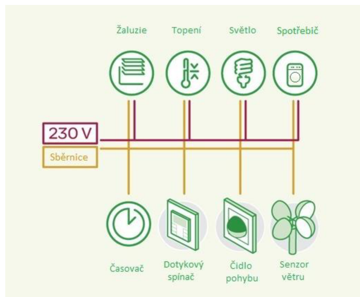
Obrázek 4-2 Systémová elektroinstalace [25]
