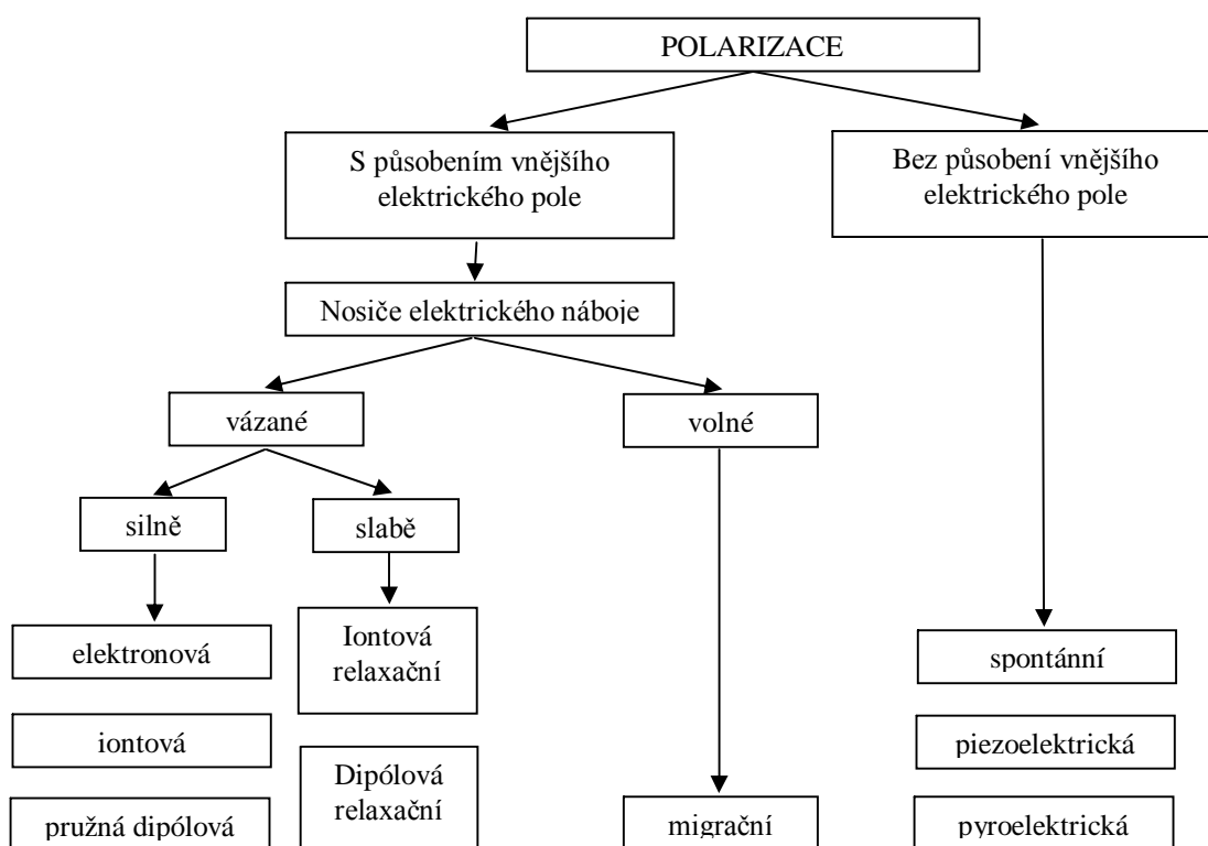
Obr. 2 Druhy polarizačních mechanismů
