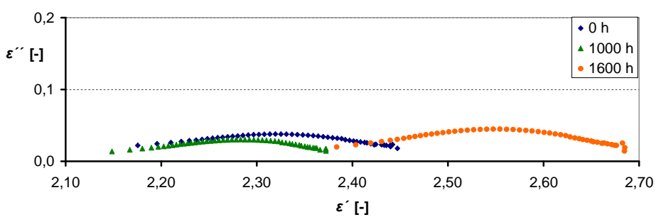
Obr. 11 Závislost \epsilon' = F(f) , \epsilon'' = F(f) a Coleho-Coleho kruhový diagram při teplotě 20 °C (teplota stárnutí 220 °C)
