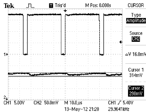
Obr. 7.4: Zvlnenie prúdu na tlmivke pri s = 0,88
