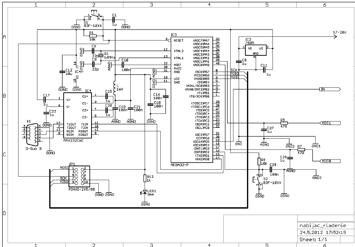
Obr. 6.2: Schéma zapojenia nabíjača, riadiaca časť
