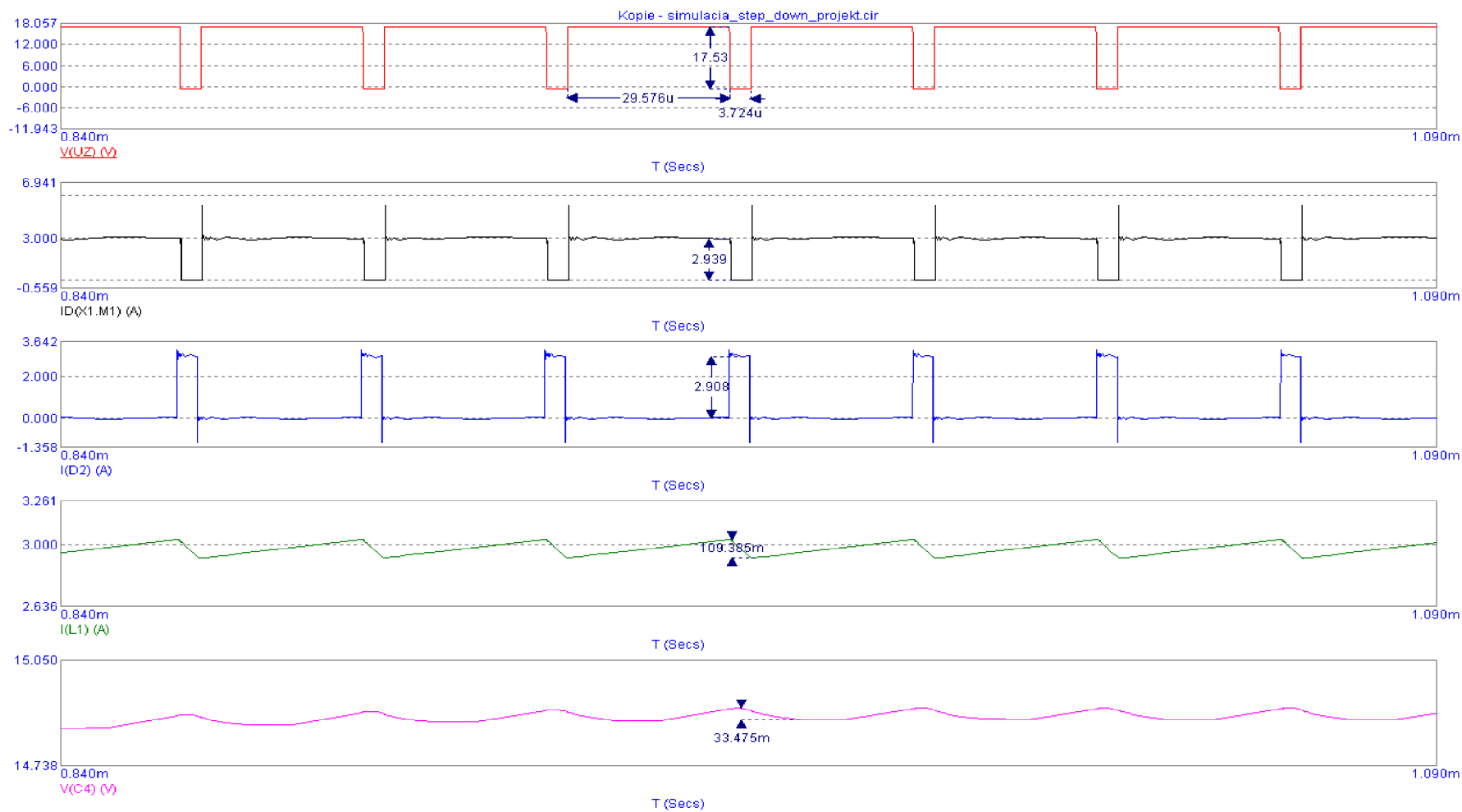
Obr. 5.6: Priebehy na meniči s výstupným napätím 15 V a zaťažovacím prúdom 3 A
