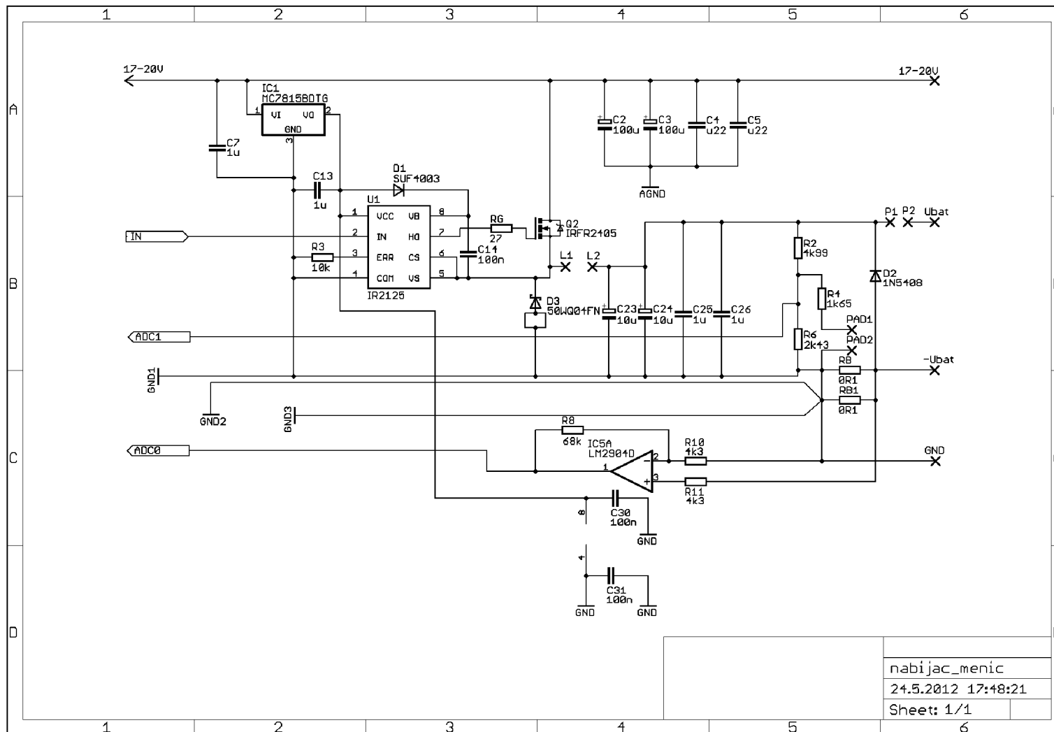
Obr. 6.1: Schéma zapojenia nabíjača, výkonová časť
