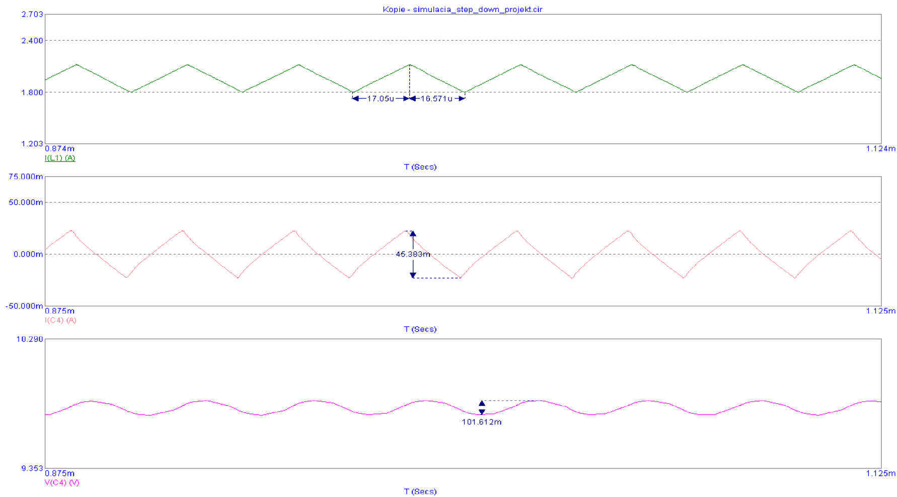
Obr. 5.3: Priebeh prúdu a napätia na výstupnom kondenzátore
