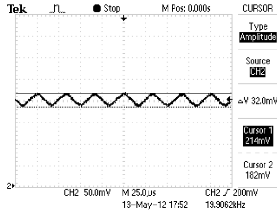
Obr. 7.3: Zvlnenie prúdu na tlmivke pri s = 0,5
