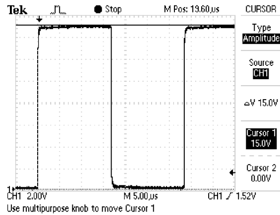
Obr. 7.6: Výstupné impulzy budiča
