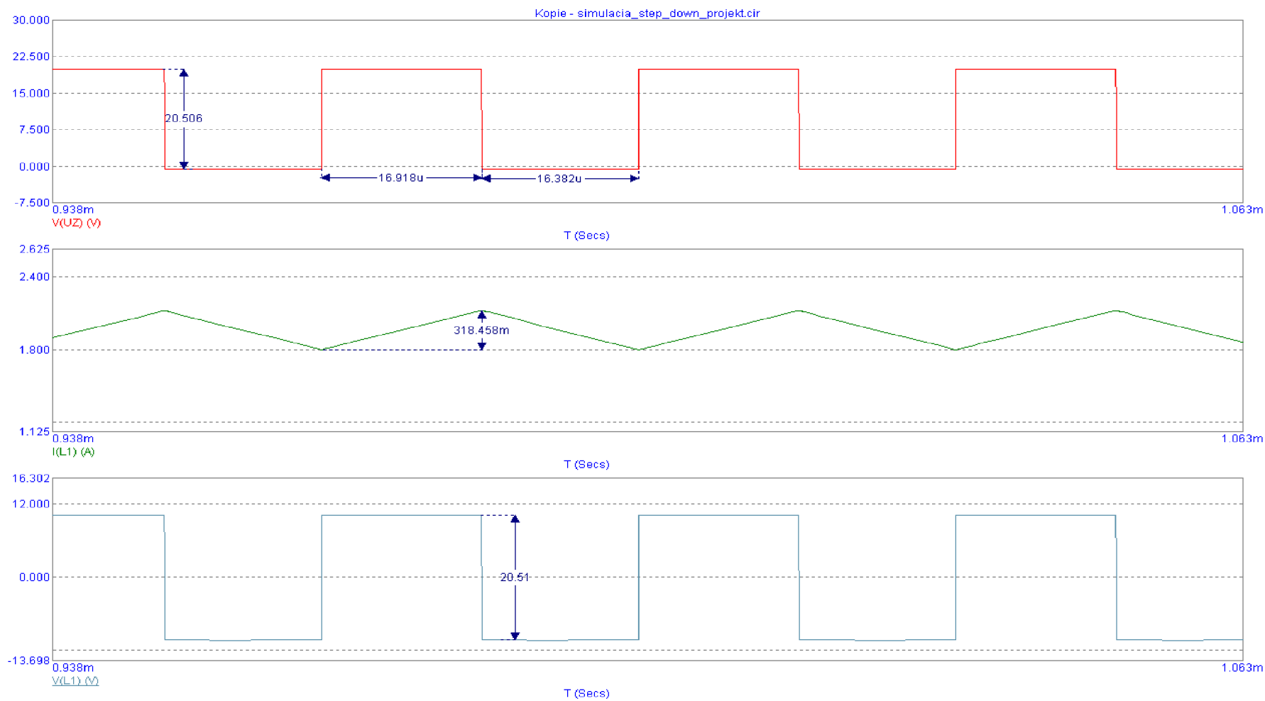
Obr. 5.2: Priebeh zvlneného prúdu a napätia na výstupnej tlmivke
