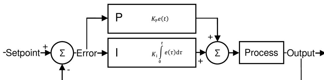
Obr. 9.2: PI regulátor
