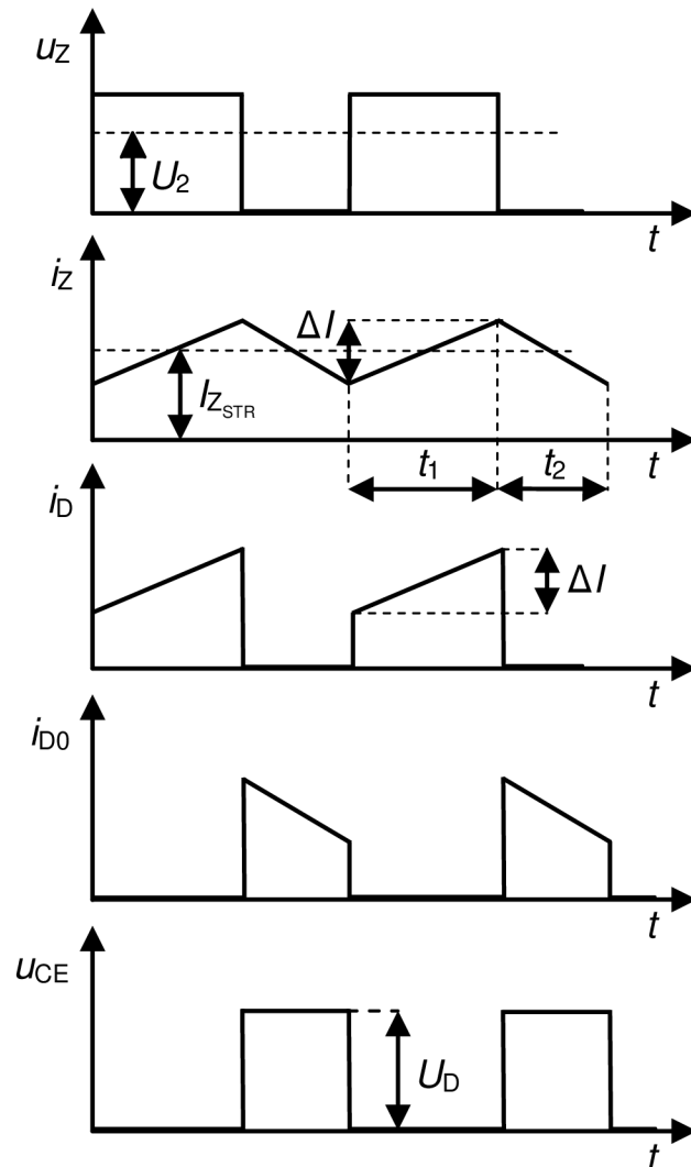
Obr. 3.2: Priebehy na jednotlivých prvkoch meniča
