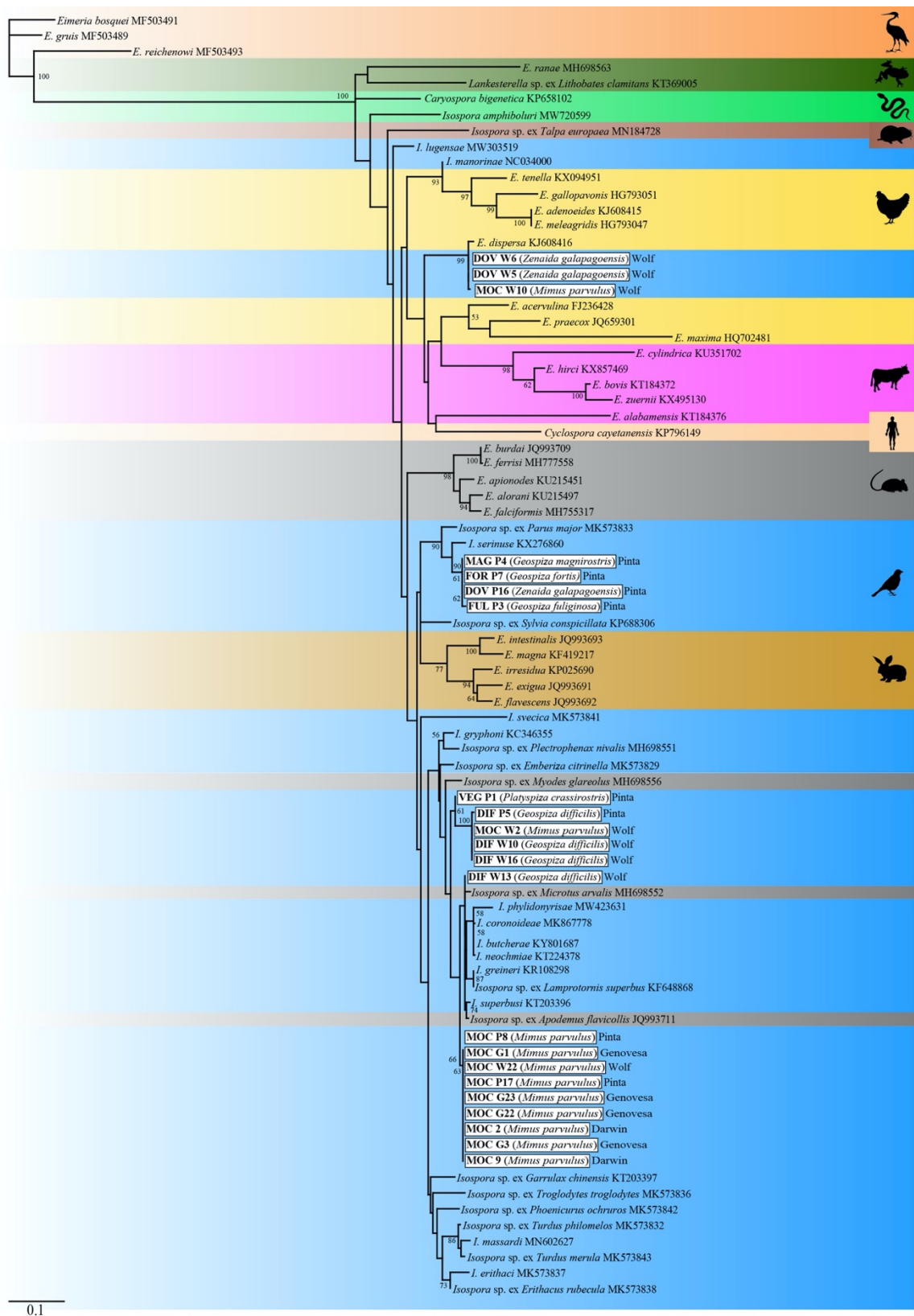
Obr. 13 Fylogenetické vztahy parazitů rodu Eimeria a Isospora rekonstruované ML analýzou sekvencí genu COI s parametry uvedenými v Tab. 1. Číselná hodnota u uzlů odpovídá bootstrapovým hodnotám (hodnoty nižší než 50 % nejsou uvedeny). Strom je zakořeněn druhem E. bosquei . Sekvence získané v rámci této práce jsou označeny bílými rámečky.
