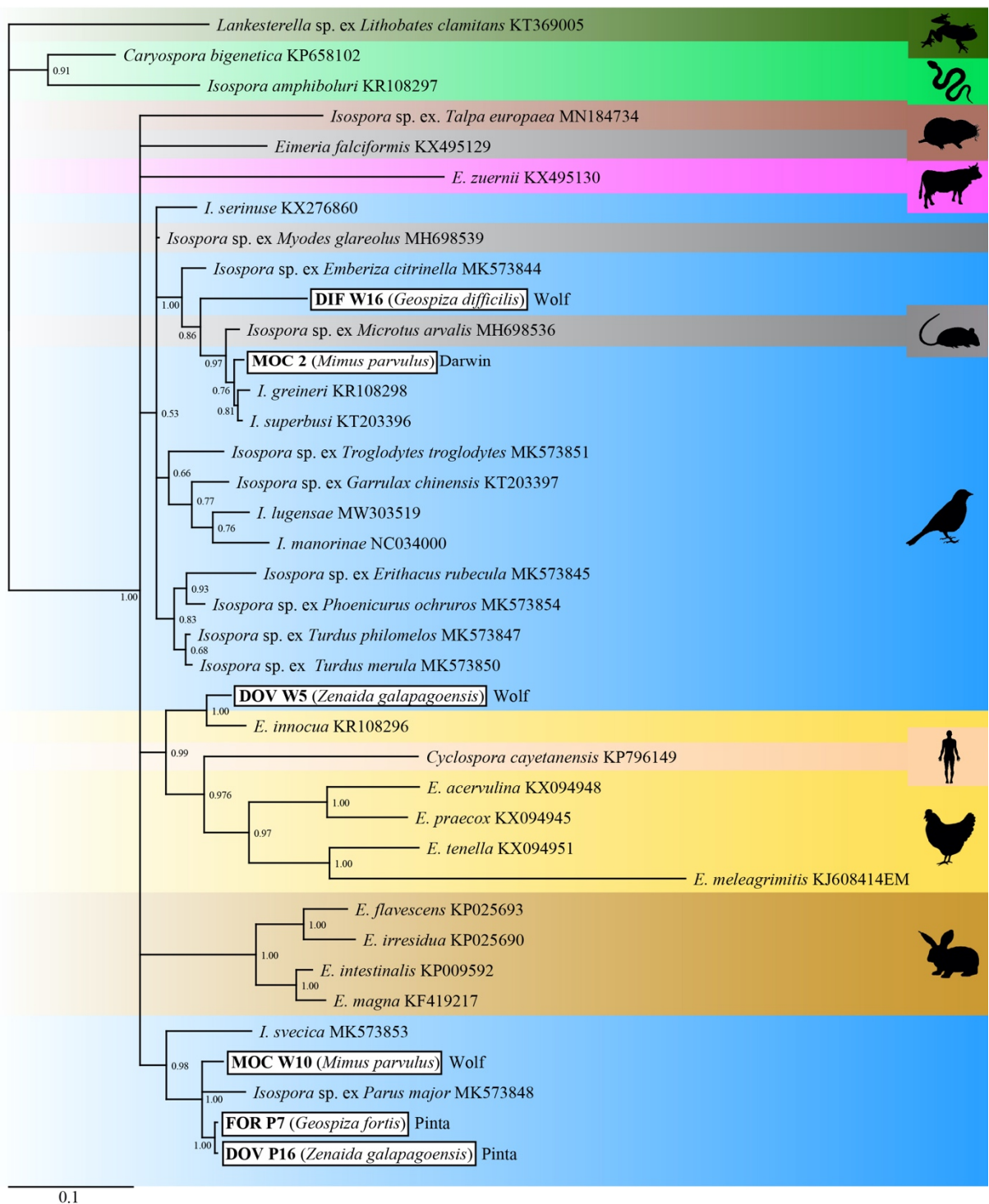
Obr. 12 Fylogenetické vztahy parazitů rodu Eimeria a Ispora rekonstruované BI analýzou sekvencí genu COIII s parametry uvedenými v Tab. 1. Číselná hodnota u uzlů odpovídá hodnotám posteriorní pravděpodobnosti (hodnoty nižší než 0,50 nejsou uvedeny). Strom je zakořeněn Lankesterella sp. Sekvence získané v rámci této práce jsou označeny bílými rámečky.
