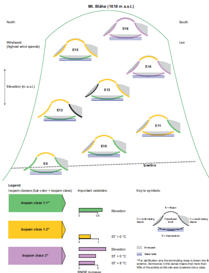
Obrázek: 6: Zobrazení stanovištního rozmístění druhových skupin podle výškových gradientů na Mt. Blåhe. V každém gradientu je podle barvy (zelená 1.1, žlutá 1.2 a fialová 2.) zobrazen výskyt dominantních stanovištních skupin v jednotlivých topografických polohách: hřebeny, prohlubně, severní návětrné svahy(vlevo) a jižní svahy(vpravo). Pro objasnění prostorového rozmístění byla pro každé místo stanovena dominantní skupina s více než 50 % aktivity. Příčná čára dole označuje horní hranici lesa. Zdroj: BECKERS et al. 2018.
