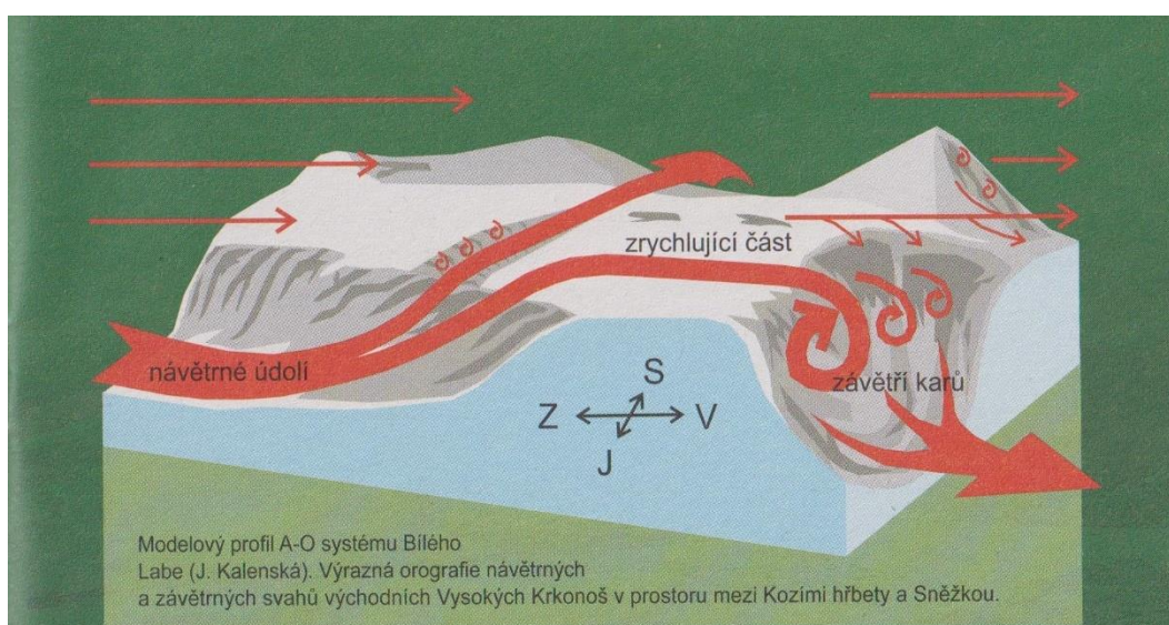
Obrázek 12: Anemo-orografický systém východních Krkonoš. Zdroj: KOCIÁNOVÁ et al. 2015
