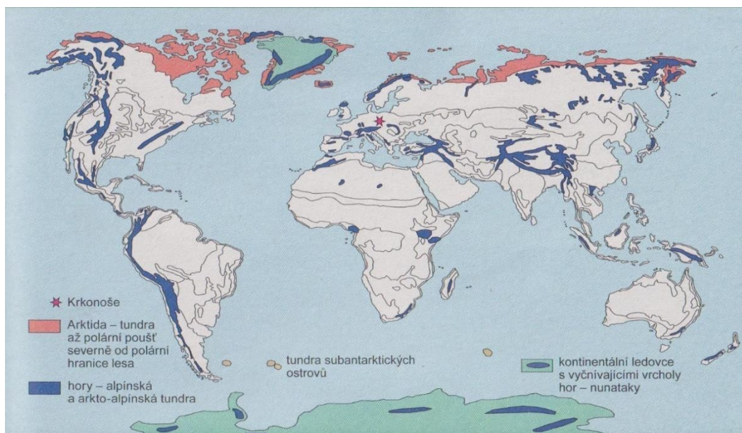
Obrázek 1: Rozšíření tundrového biomu na Zemi. Rozšíření alpské tundry (modrá barva) převažuje na severní polokouli. Zdroj: Kociánová et al. 2015
