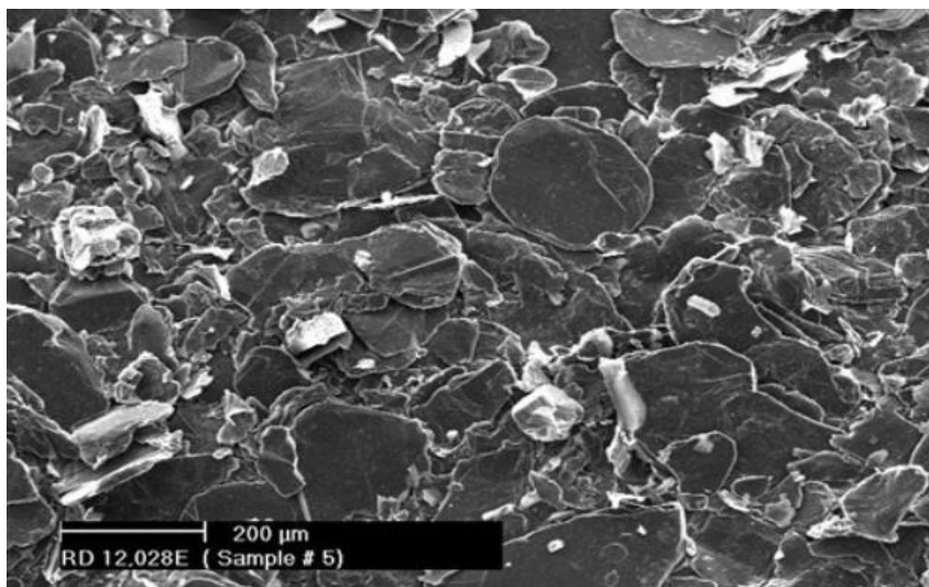
Obrázek 2.2: SEM snímek povrchu vločkového grafitu. [18]
