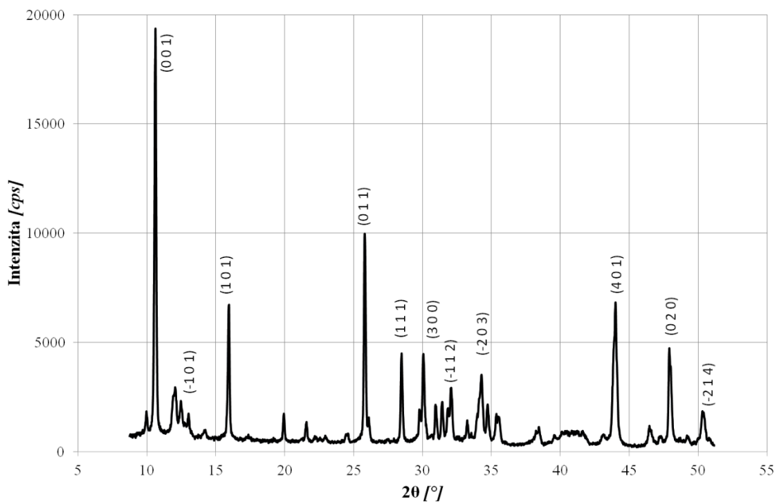
Obrázek 7.2: XRD spektrum pro vzorek 1c včetně orientace pro fázi \text{Na}_2\text{Ti}_3\text{O}_7 .
