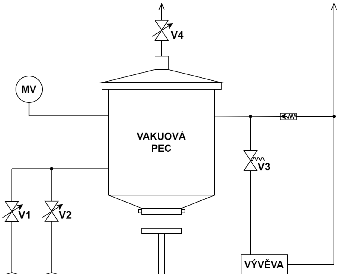
Obrázek 5.2: Konceptní schéma vakuové pece. [převzato ze štítku pece]
