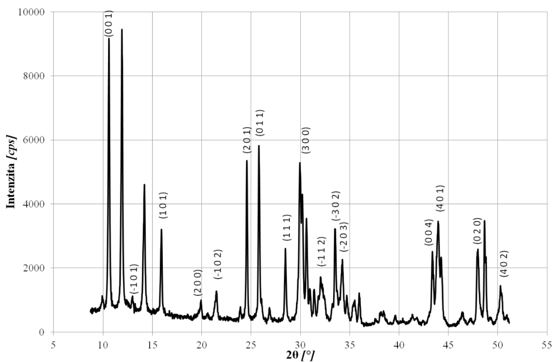
Obrázek 7.3: XRD spektrum pro vzorek 2a včetně orientace pro fázi \text{Na}_2\text{Ti}_3\text{O}_7 .
