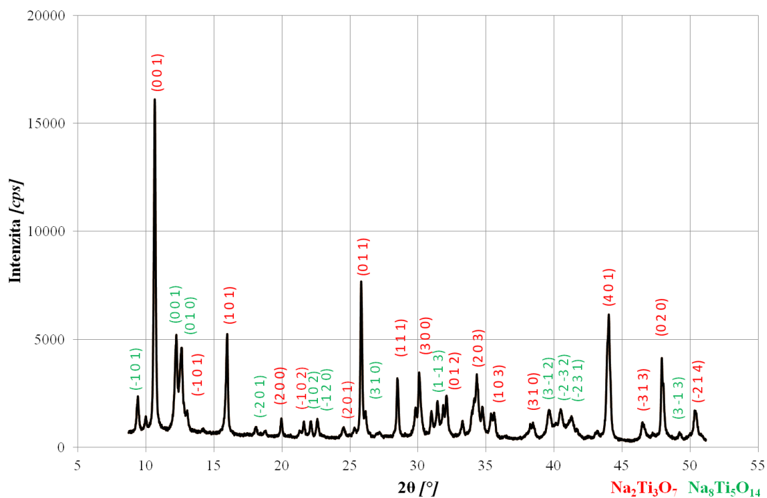
Obrázek 7.5: XRD spektrum pro vzorek 4a včetně orientací pro fázi Na 2 Ti 3 O 7 (červená barva) a pro fázi Na 8 Ti 5 O 14 (zelená barva).
