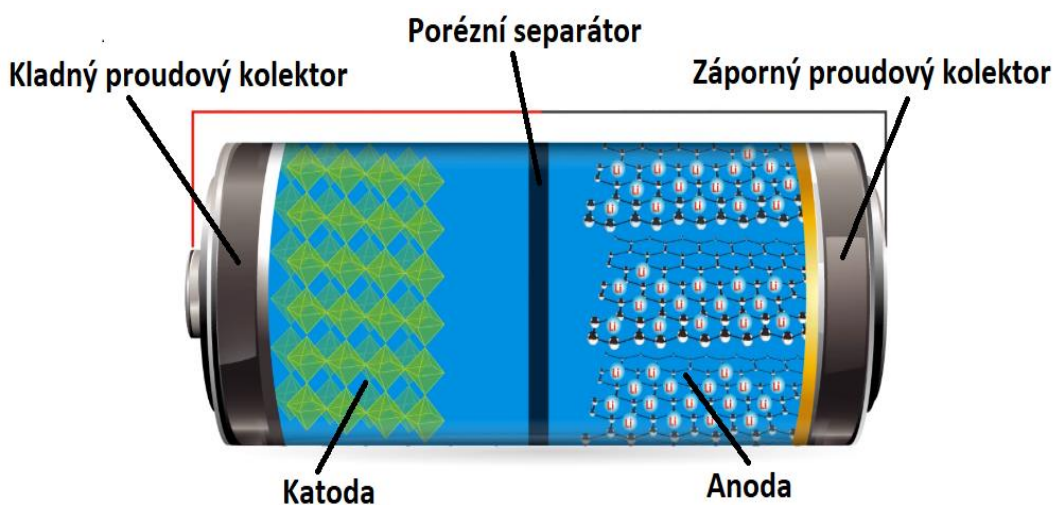
Obrázek 2.1: Zobrazení základních částí lithium-ionového akumulátoru. [8]
