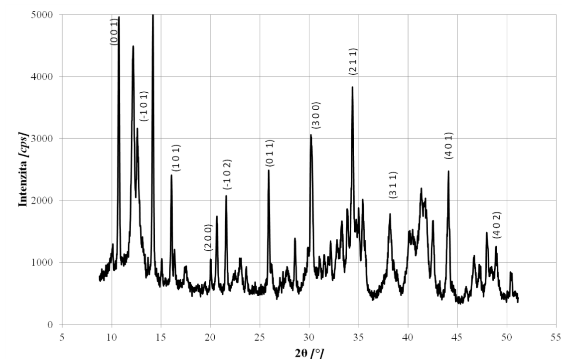
Obrázek 7.4: XRD spektrum pro vzorek 3a včetně orientace pro fázi Na 2 Ti 3 O 7 .
