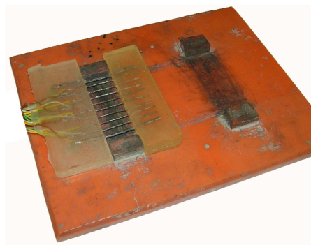
Obr. 6.5: Pastování elektrody
