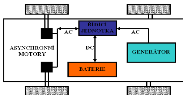
Obr. 1.2: Princip sériové koncepce hybridního automobilu
