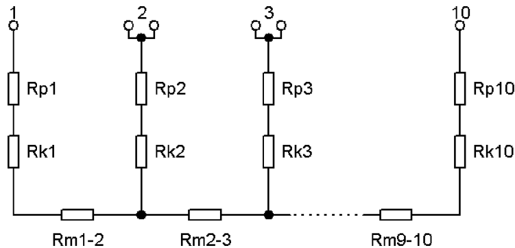
Obr. 5.3: Náhradní schéma elektrody s kolektorem s nespojitým systémem rovnoběžných žebor
