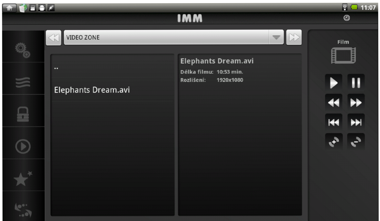
Obrázek 4.9: Aktivita VideoActivity.
