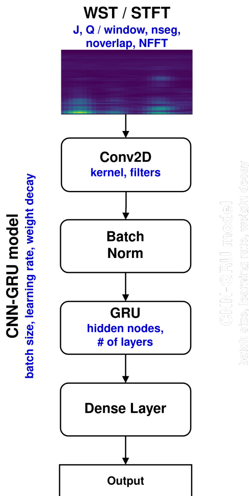
Fig. 5.3: CNN-GRU model with highlighted optimizable parameters in blue
