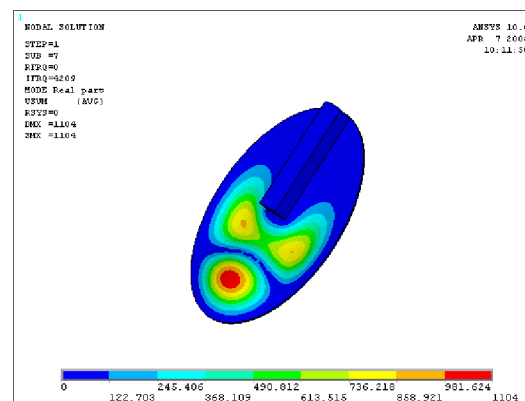
Obr. 4.1 První čtyři tvary kmitu bubínku pro úhel 50^\circ
