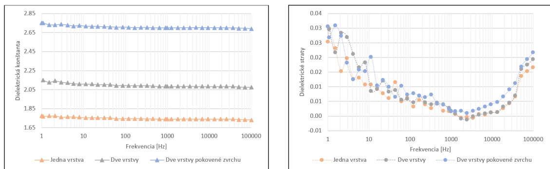
Obr. 4.12: Graf závislosti dielektrickej konštanty a dielektrických strát vzorky 40-01 pokovenej hliníkovým práškom na frekvencii.
