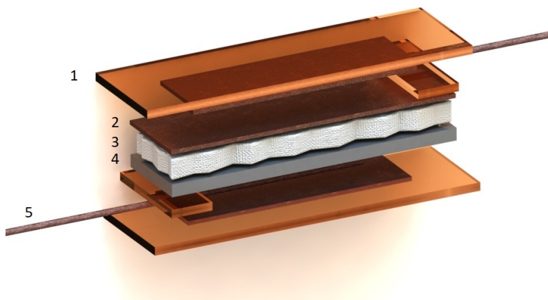
Obr. 5.1: Model senzorského zariadenia zo softvéru SolidWorks. Jednotlivé materiály: 1 - kaptónový film, 2 - medená páska, 3 - nanovláknenná maticu, 4 - hliníkový alobal, 5 - medený drôt ako elektróda.
