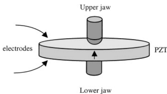
Obr. 4.5: Geometria vzorky vo svorkách d_{33} metra [28].
