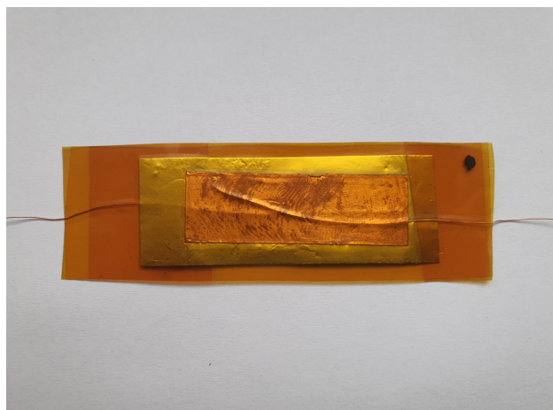
Obr. 5.2: Výsledné experimentálne senzorické zariadenie.
