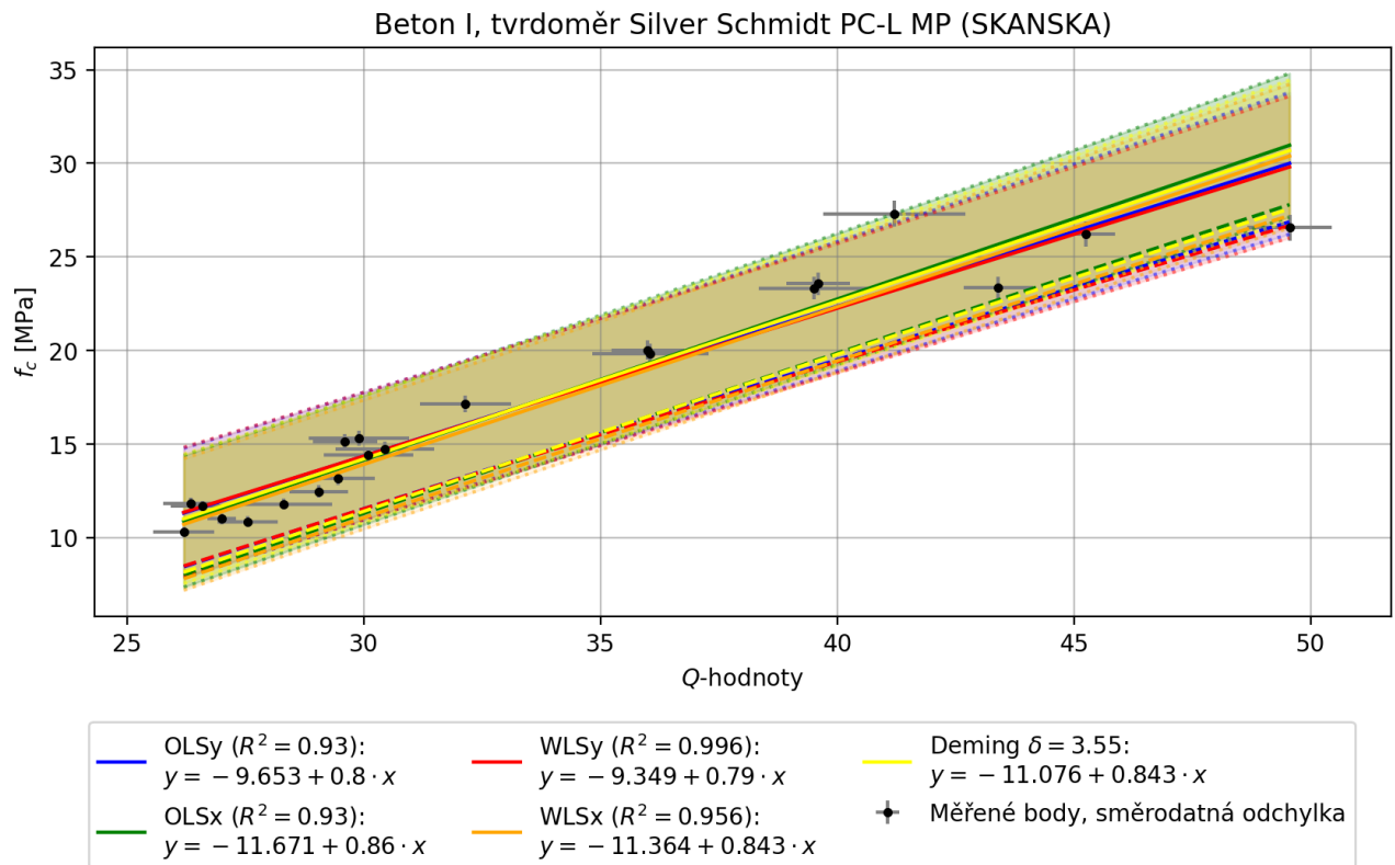
Obr. 36: Data 2: výsledné regresní křivky a spolehlivostní pásy pro beton I, tvrdoměr SilverSchmidt PC-L MP (SKANSKA).
