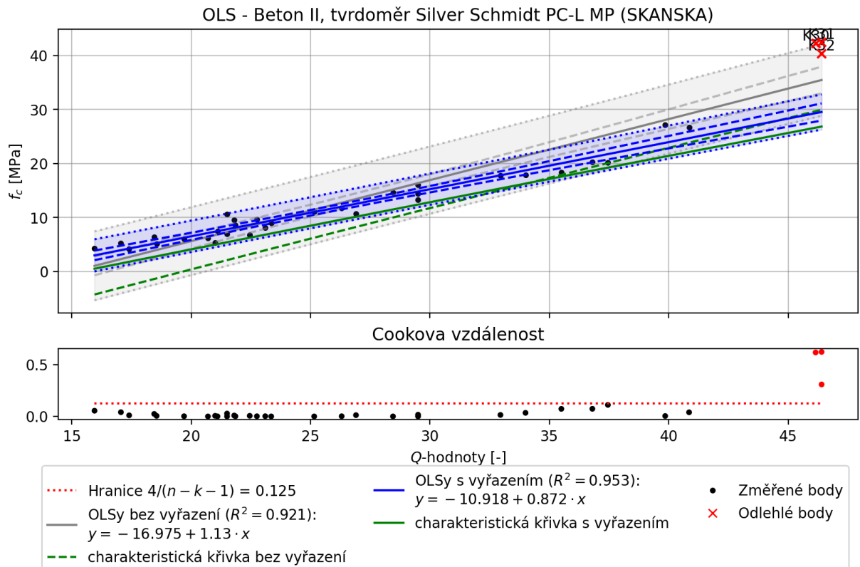
Obr. 46: Data 2: vykreslení Cookovy vzdálenosti regresní křivky před vyřazením identifikovaných odlehých bodů a po vyřazení. Beton II, tvrdoměr SilverSchmidt PC-L MP (SKANSKA).
