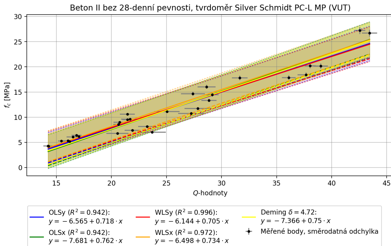
Obr. 41: Data 2: výsledné regresní křivky a spolehlivostní pásy pro beton II s vyřazením 28-denní pevnosti, tvrdoměr SilverSchmidt PC-L MP (SKANSKA).
