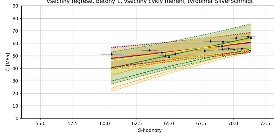
Všechny regrese, betony 1, všechny cykly měření, tvrdoměr SilverSchmidt
