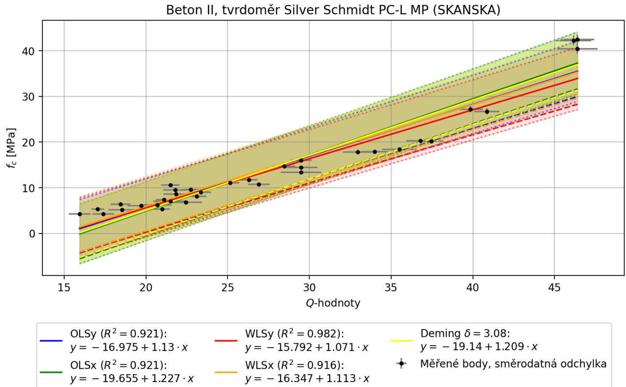
Obr. 38: Data 2: výsledné regresní křivky a spolehlivostní pásy pro beton II, tvrdoměr SilverSchmidt PC-L MP (SKANSKA).
