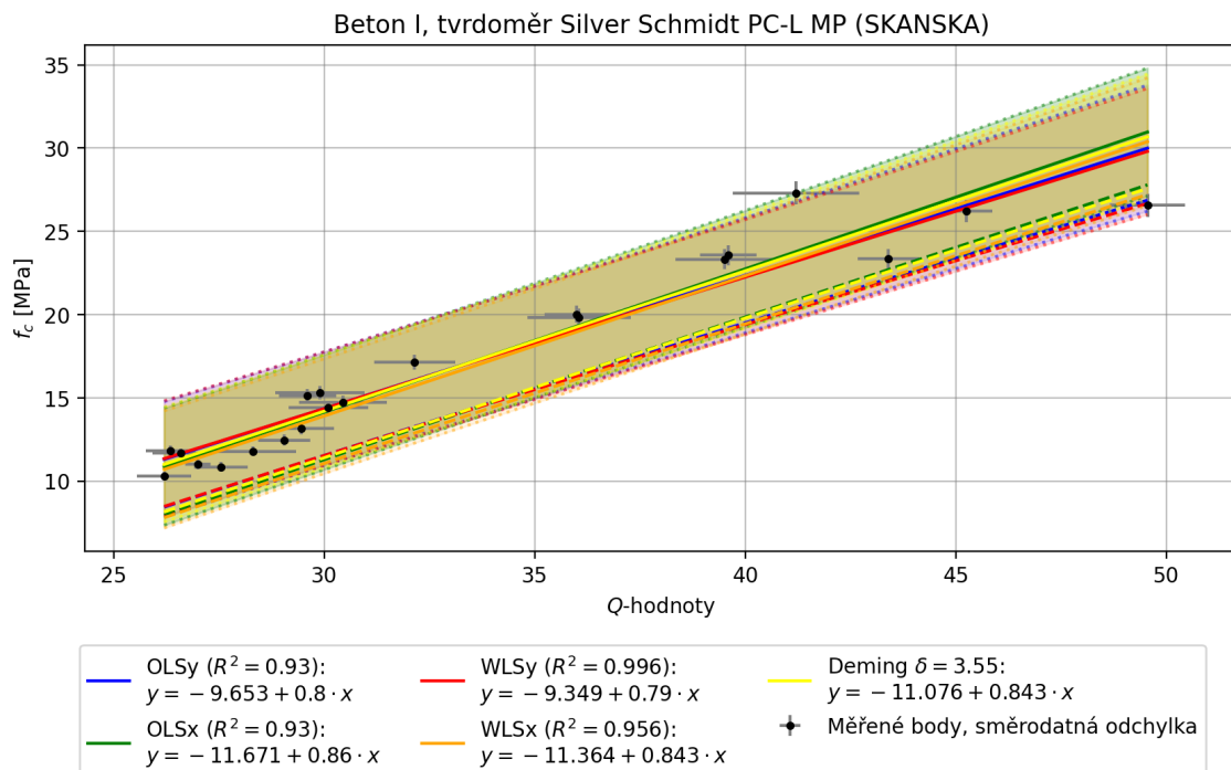
Obr. 20: Data 2: výsledné regresní křivky a spolehlivostní pásy pro beton I, tvrdoměr Silver-Schmidt PC-L MP (SKANSKA).
