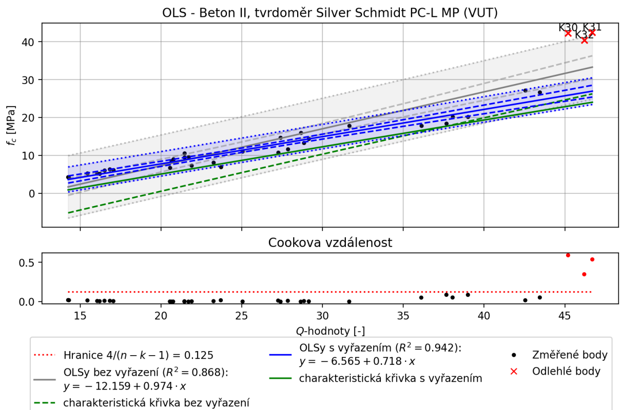
Obr. 47: Data 2: vykreslení Cookovy vzdálenosti regresní křivky před vyřazením identifikovaných odlehých bodů a po vyřazení. Beton II, tvrdoměr SilverSchmidt PC-L MP (VUT).
