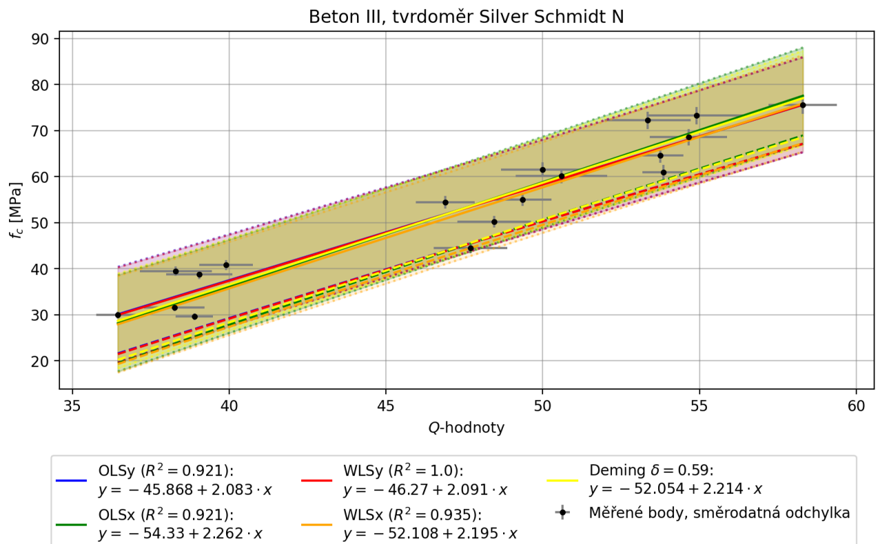
Obr. 43: Data 2: výsledné regresní křivky a spolehlivostní pásy pro beton III, tvrdoměr SilverSchmidt N.
