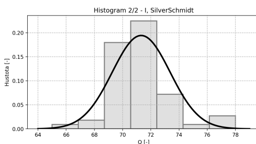
Obr. 15: Histogram hodnot vrácené energie Q bloku 2/2 - I.
