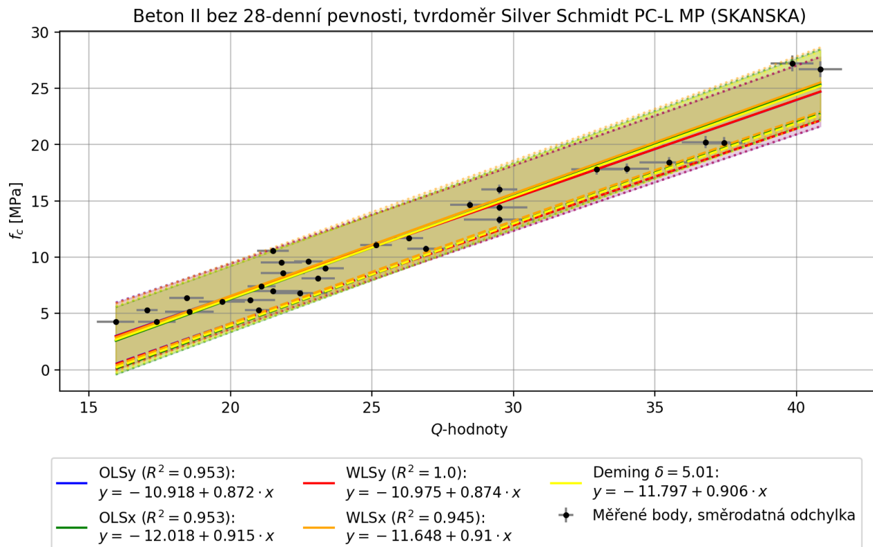
Obr. 40: Data 2: výsledné regresní křivky a spolehlivostní pásy pro beton II s vyřazením 28-denní pevnosti, tvrdoměr SilverSchmidt PC-L MP (SKANSKA).
