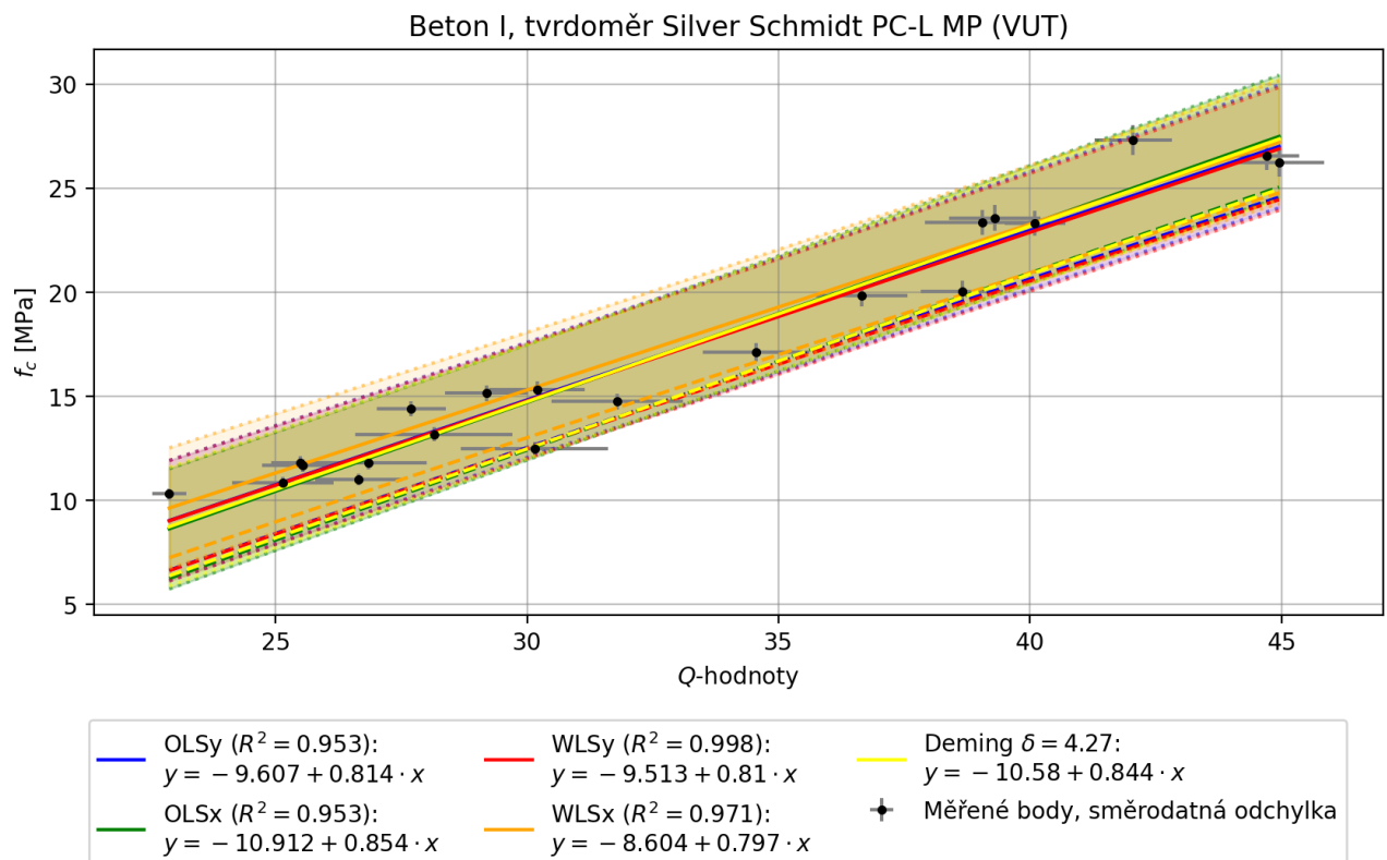
Obr. 37: Data 2: výsledné regresní křivky a spolehlivostní pásy pro beton I, tvrdoměr SilverSchmidt PC-L MP (VUT).
