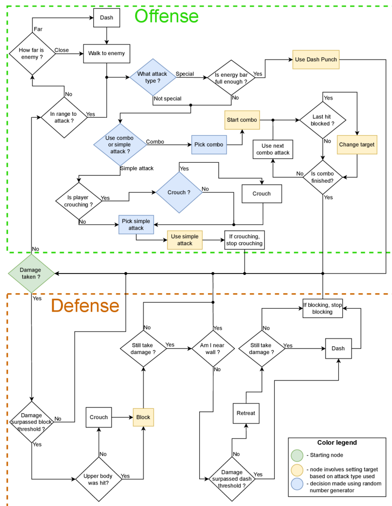
Obrázek A.1: Diagram popisující rozhodování AI. Určité aspekty rozhodování nebyly zahrnuté z důvodu přehlednosti diagramu.
