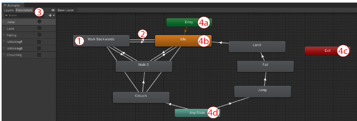
Obrázek 2.5: UI Animatora. 1. Stav reprezentujúci klip animácie. 2. Prechod medzi jednotlivými klipmi. 3. Parametre podľa ktorých sa prechody rozhodujú. 4. Špeciálne stavy, ktoré sú unikátne: a - začiatkový stav automatu, b - stav do ktorého automat vždy prejde zo stavu Entry, c - konečný stav automatu, d - stav, ktorý symbolizuje prechod z ktoréhokoľvek stavu.
