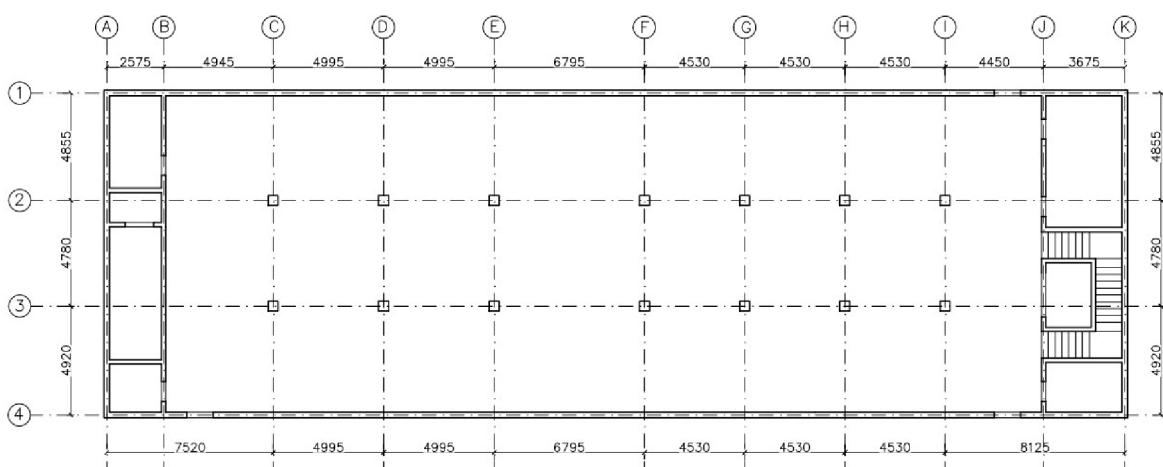
Obr. 1 schéma půdorysu objektu
