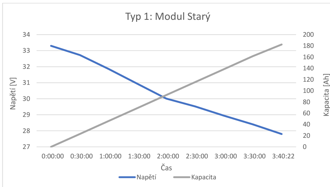
Graf. 8 Vybíjecí charakteristika: Typ 1, starý modul
