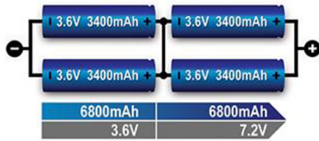
Obr. 14 Sériově paralelní zapojení čtyř článků (2s2p) [47]
