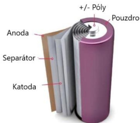
Obr. 15 Design válcového článku [48]
