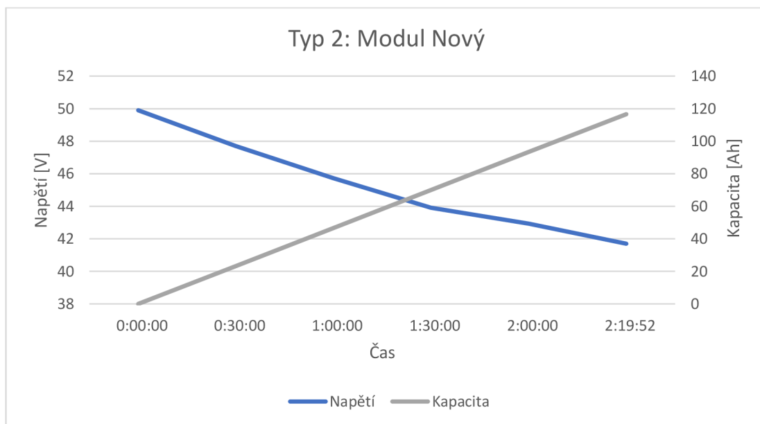
Graf. 9 Vybíjecí charakteristika: Typ 2, nový modul
