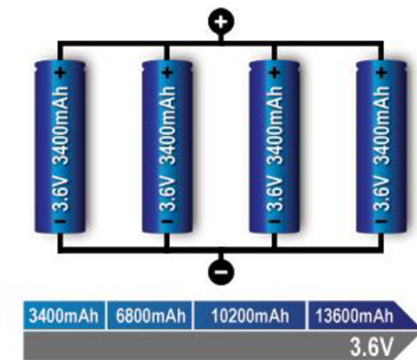
Obr. 13 Paralelní zapojení čtyř článků (4P) [47]
