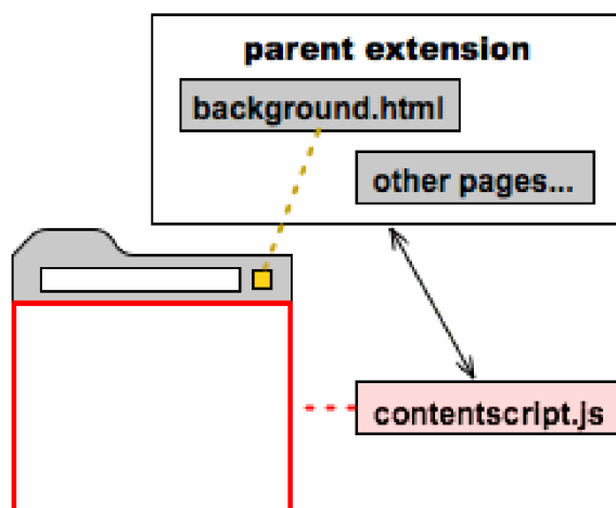
Obr. 3.4: Princíp fungovania content scriptov s background page 10
