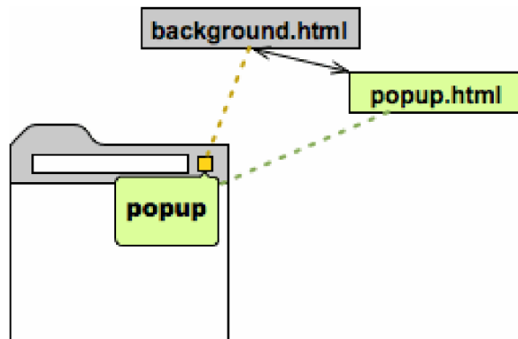
Obr. 3.3: Princíp fungovania popup okna s background page
