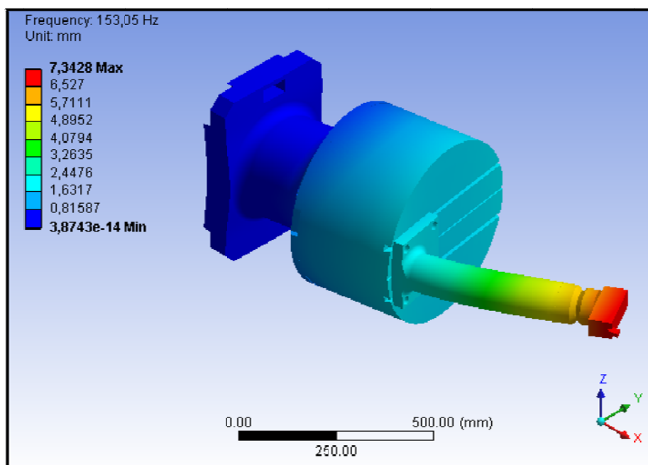
Obr. 49 Tvar kmitů – 1. mod
