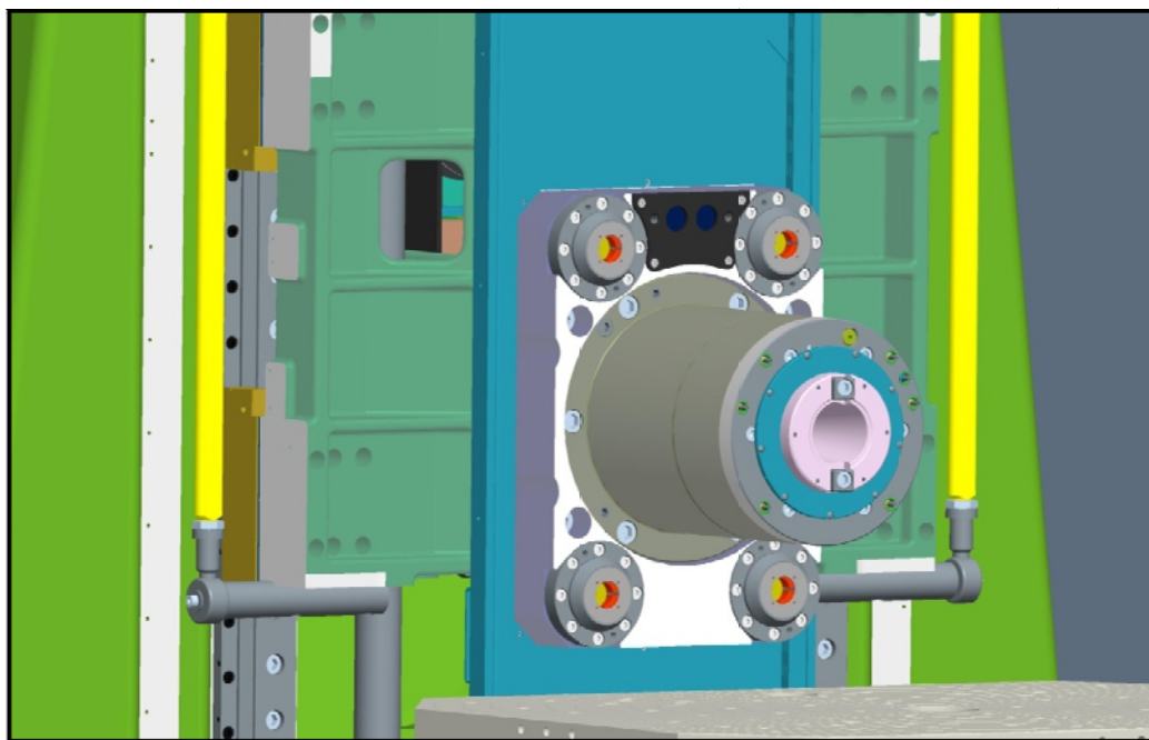
Obr. 37 Rozhraní D'Andrea upevněné na vřeteně
