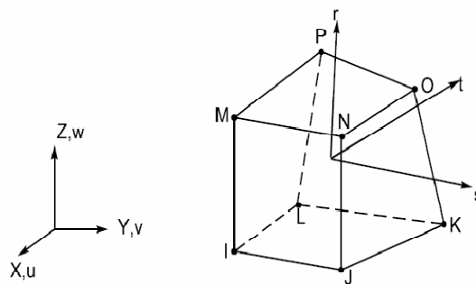
Obr. 46 Prvek SOLID185 [3]
