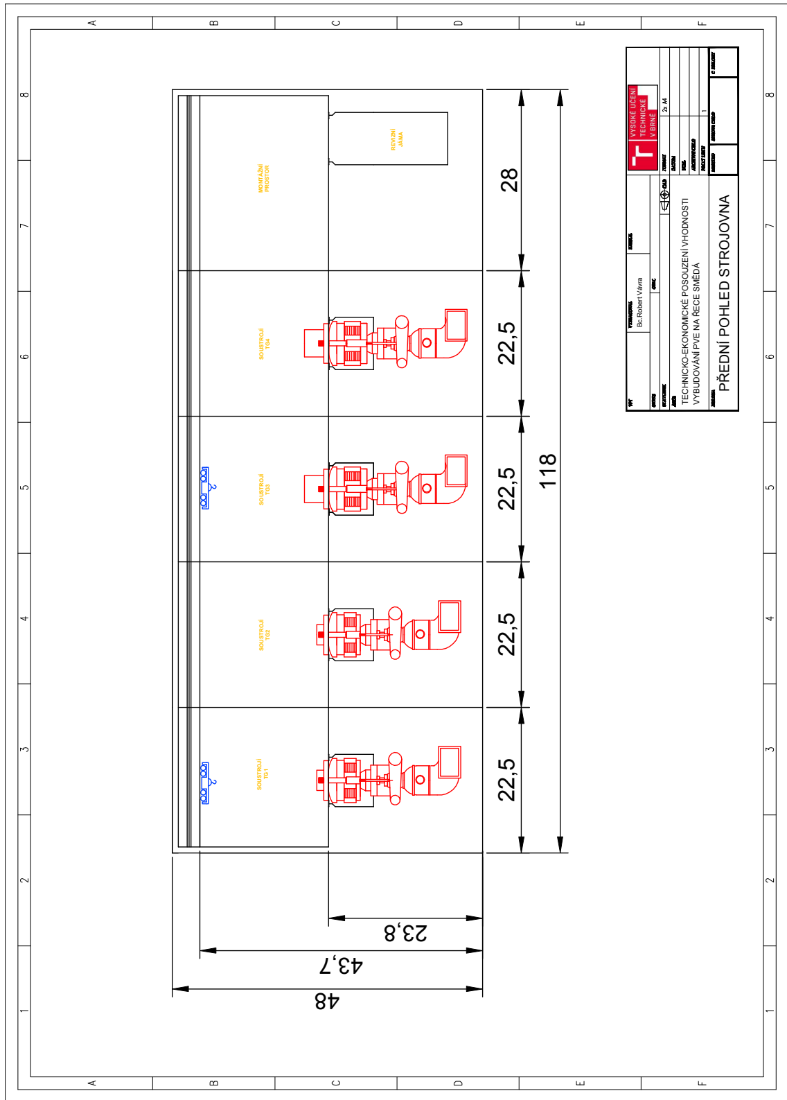
Obr. 3.6: Přední pohled strojovny
